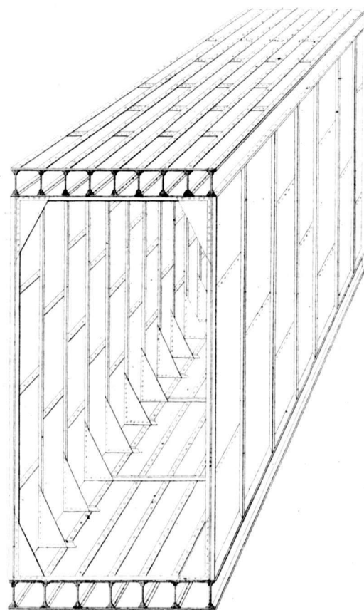
Doorsnede Fig. 3. Schaal van 1:100
