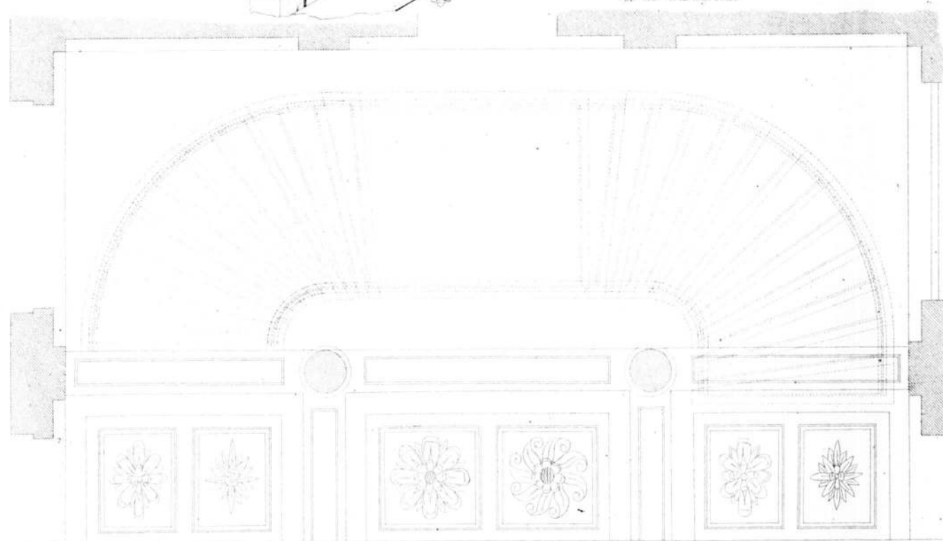
Gedeelte van de Platte grond der Vestibule en ijzeren Trap so der ware grotte.
