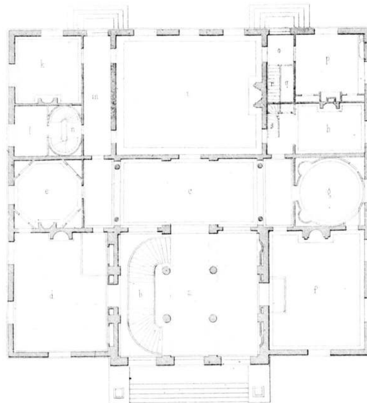
Begane grond of Rez de Chaussée
