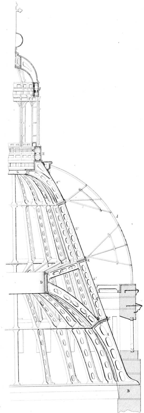
Schaal voor den Koepel
