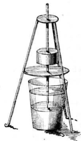
Toestel van VICAT op \frac{1}{4} .
