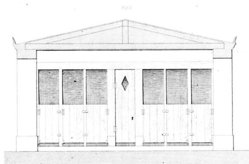
Details van de Gemakken.
