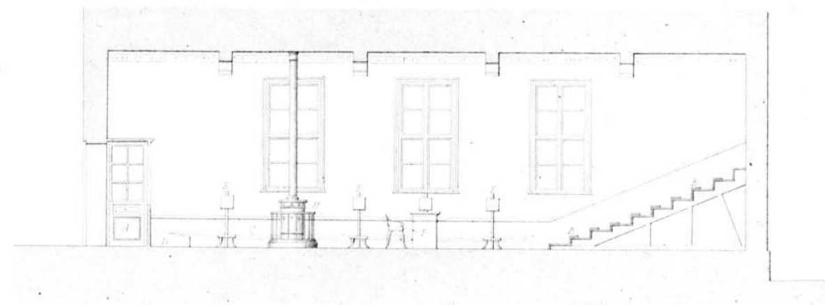
Doorsnede over de lengte der Zaal.
