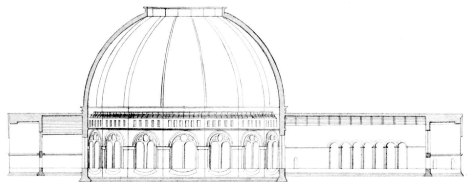
DOORSNEDE OVER DE MIDDEENZAAL OVER DE LUN AB
