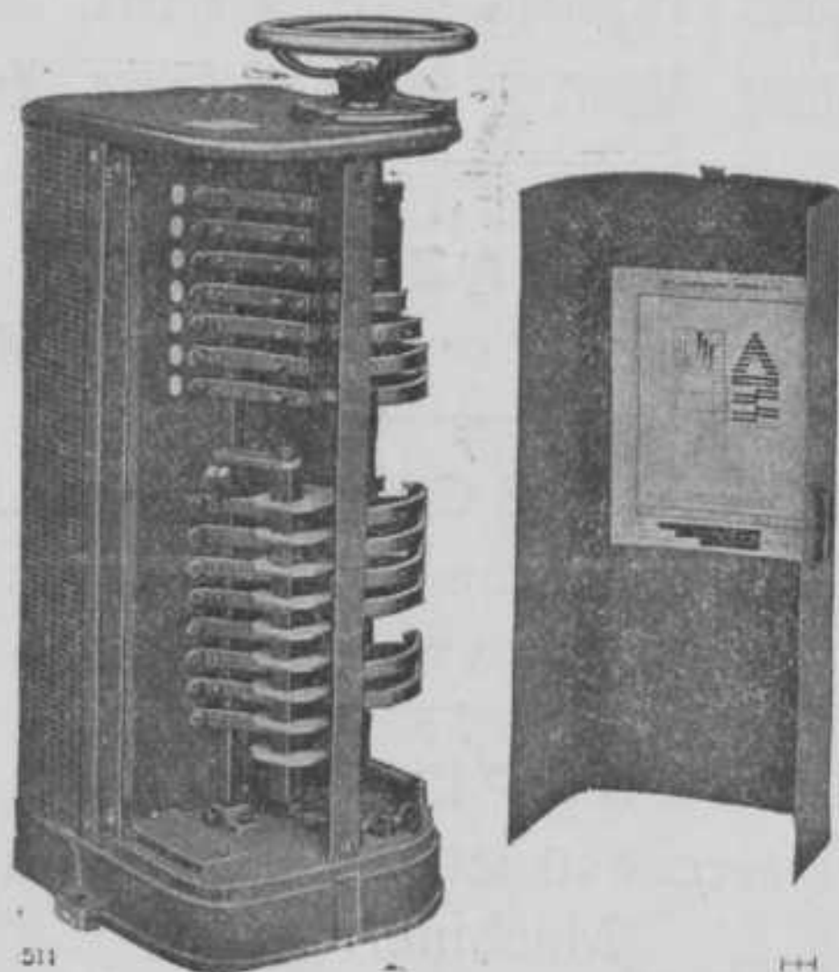
Draaistroom-omkeercontroller met aangebouwd weerstand.
