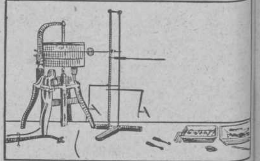
Apparaat ter bepaling van de working van verschillende vergiften op het hart.
