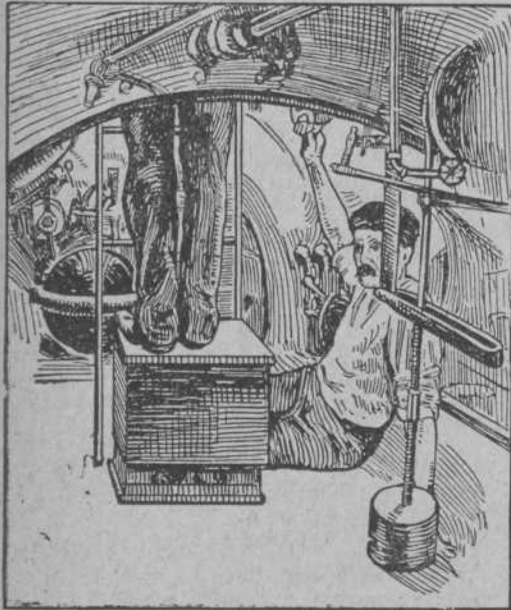
Machineruim en stuurstoel van de Amerik. onderzeeboot „Holland”. De groote slinger regelt de machinerie, die de boot op de verlangde diepte houdt.
