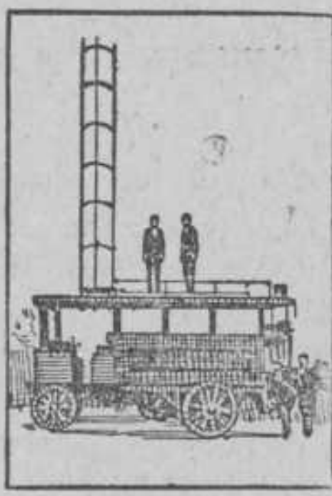
Verplaatsbaar station voor Marconi's draadloze telegraaf, gekonstrueerd op een auto.
