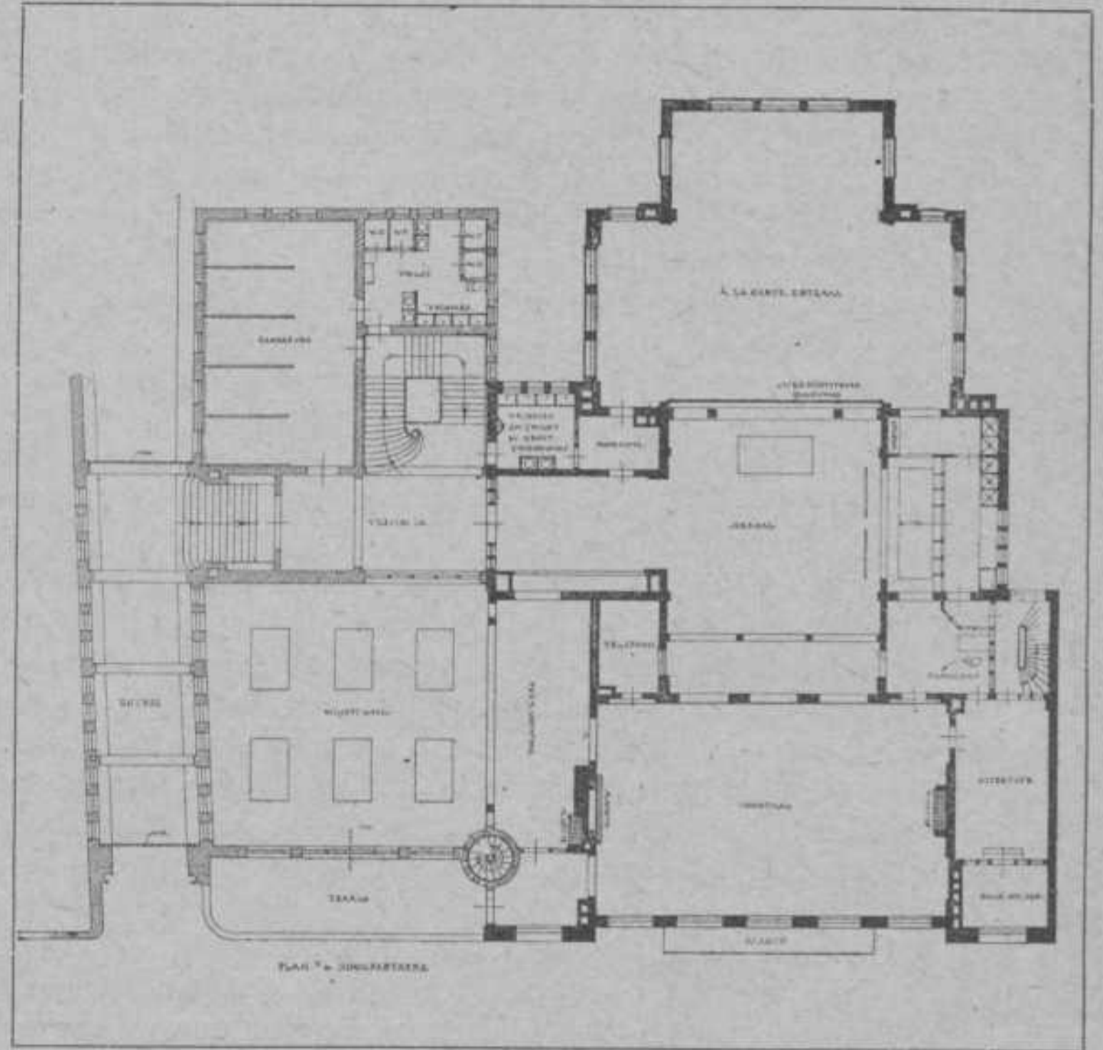
Bouwplan Van Loghem.
