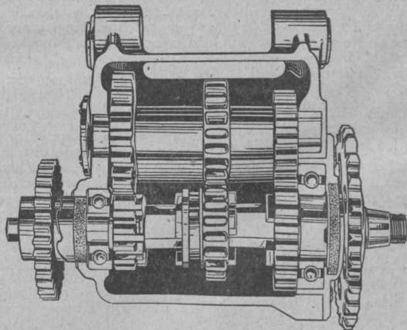
Versnellingsbak.
