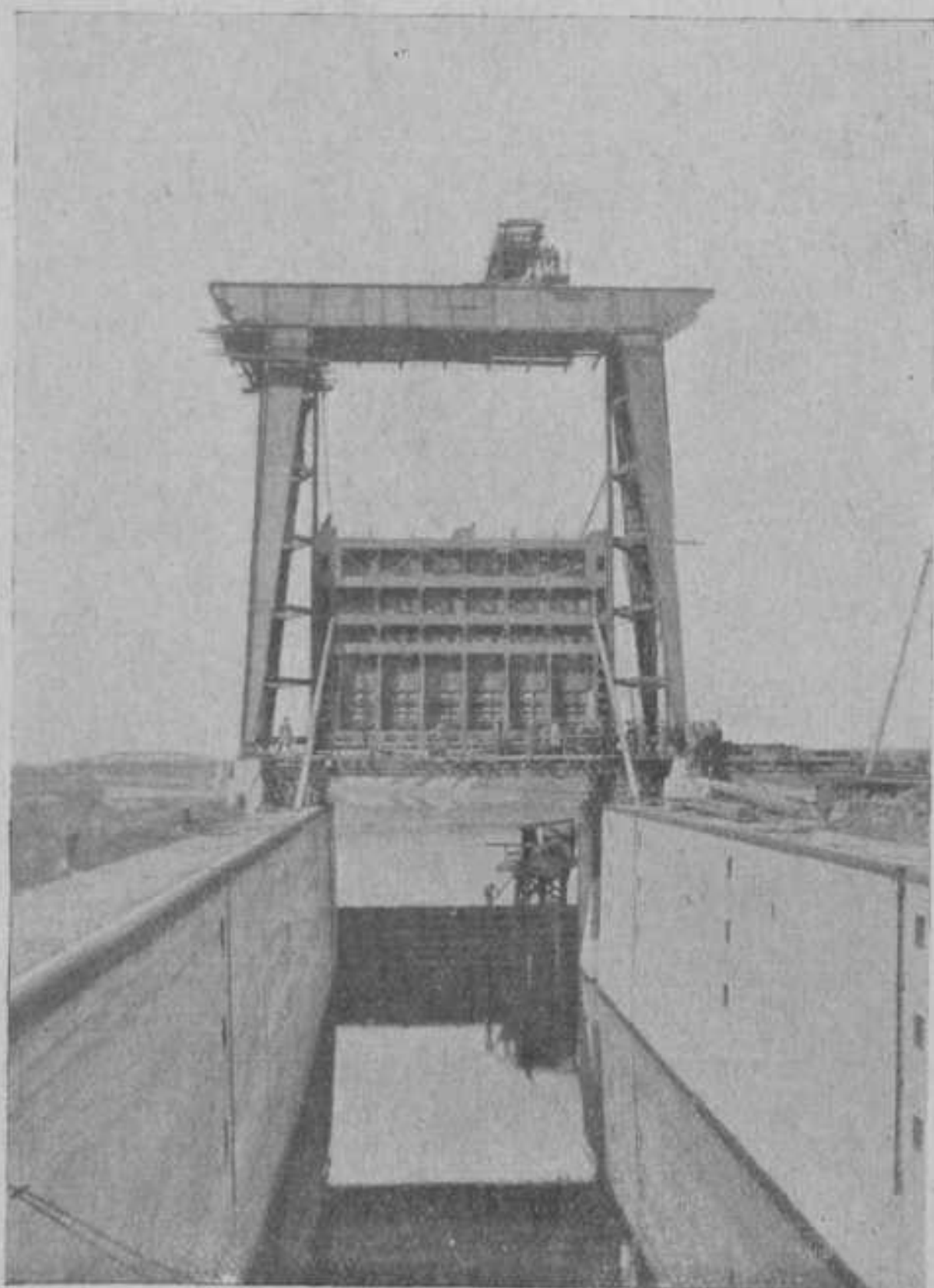
Sluis in Lippekanaal met hefdeur.
