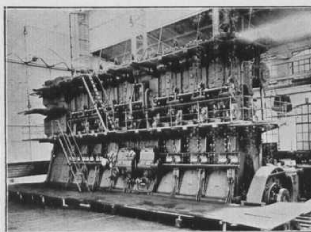
Dubbelwerkende tweetakt motor 5800 As P.K.
