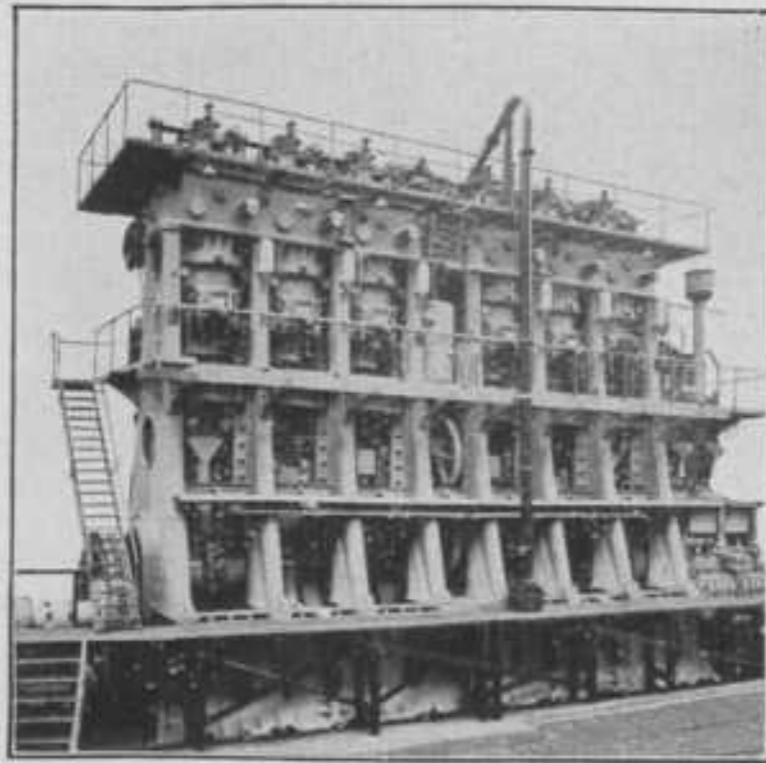
SCHEEPSDIESELMOTOREN
