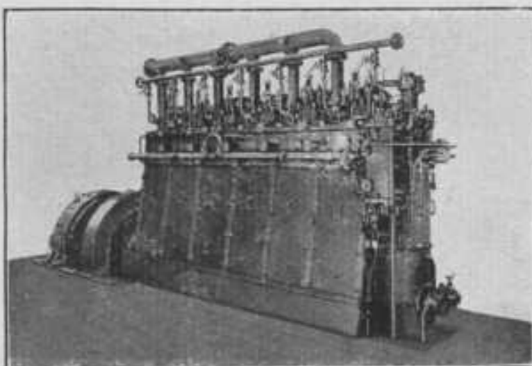
STATIONNAIRE DIESELMOTOREN
