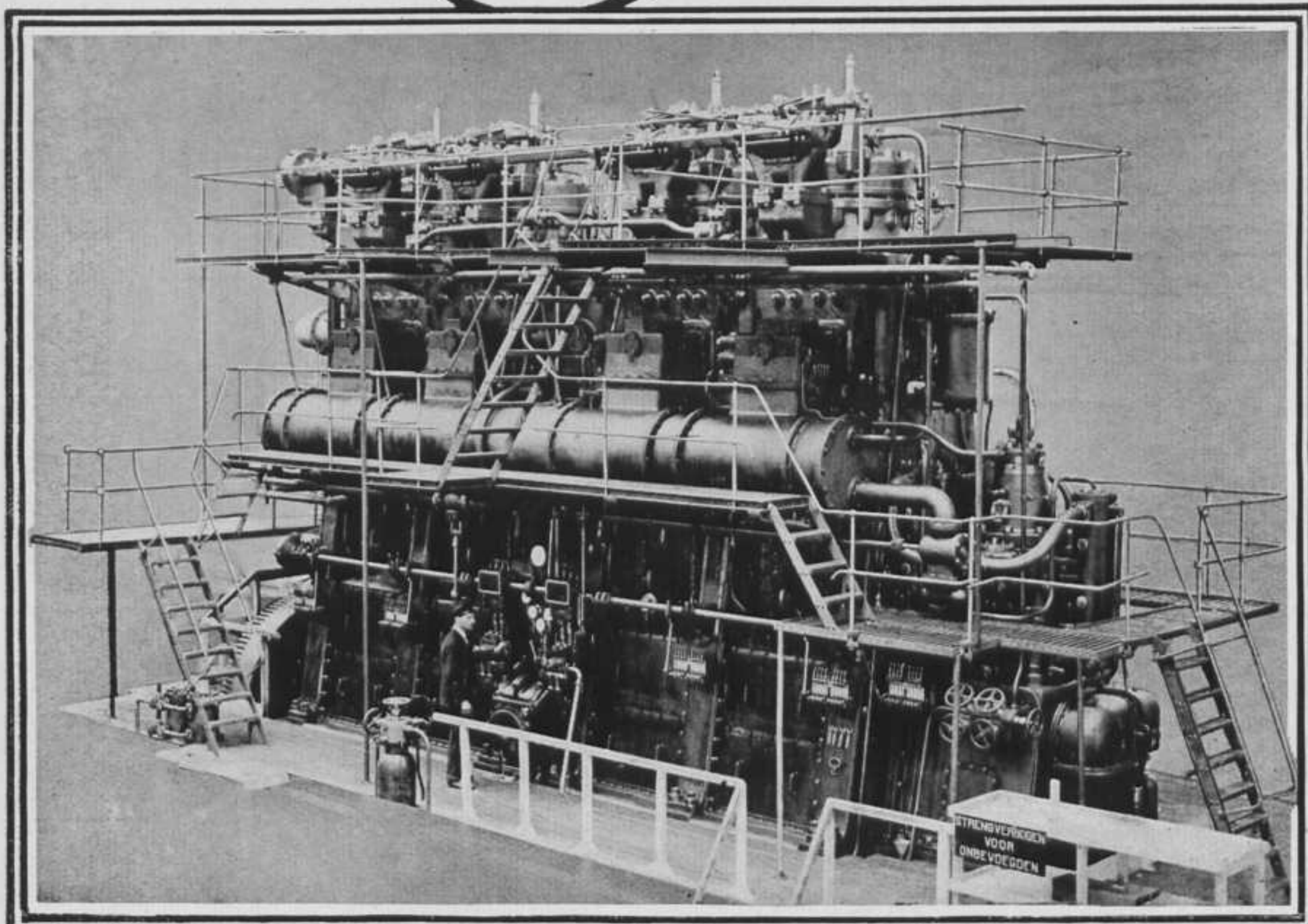
2000 A.P.K.SCHEEPS DIESEL MOTOR
