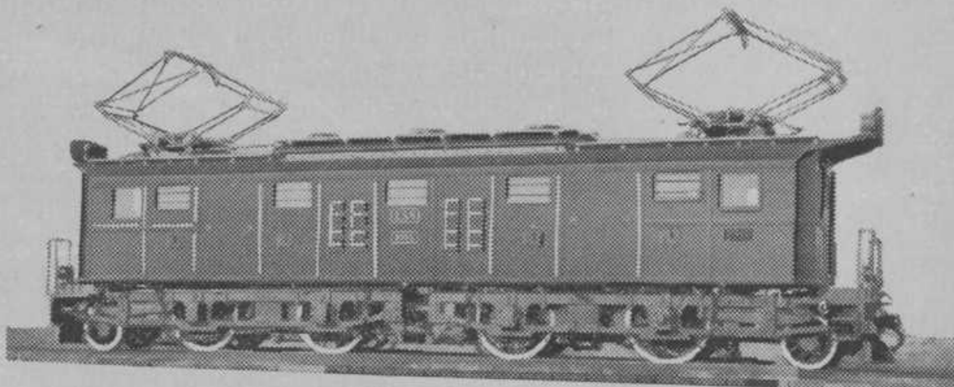
Een der 6 elektrische locomotieven 1200 pk. voor Ned. Indië.
