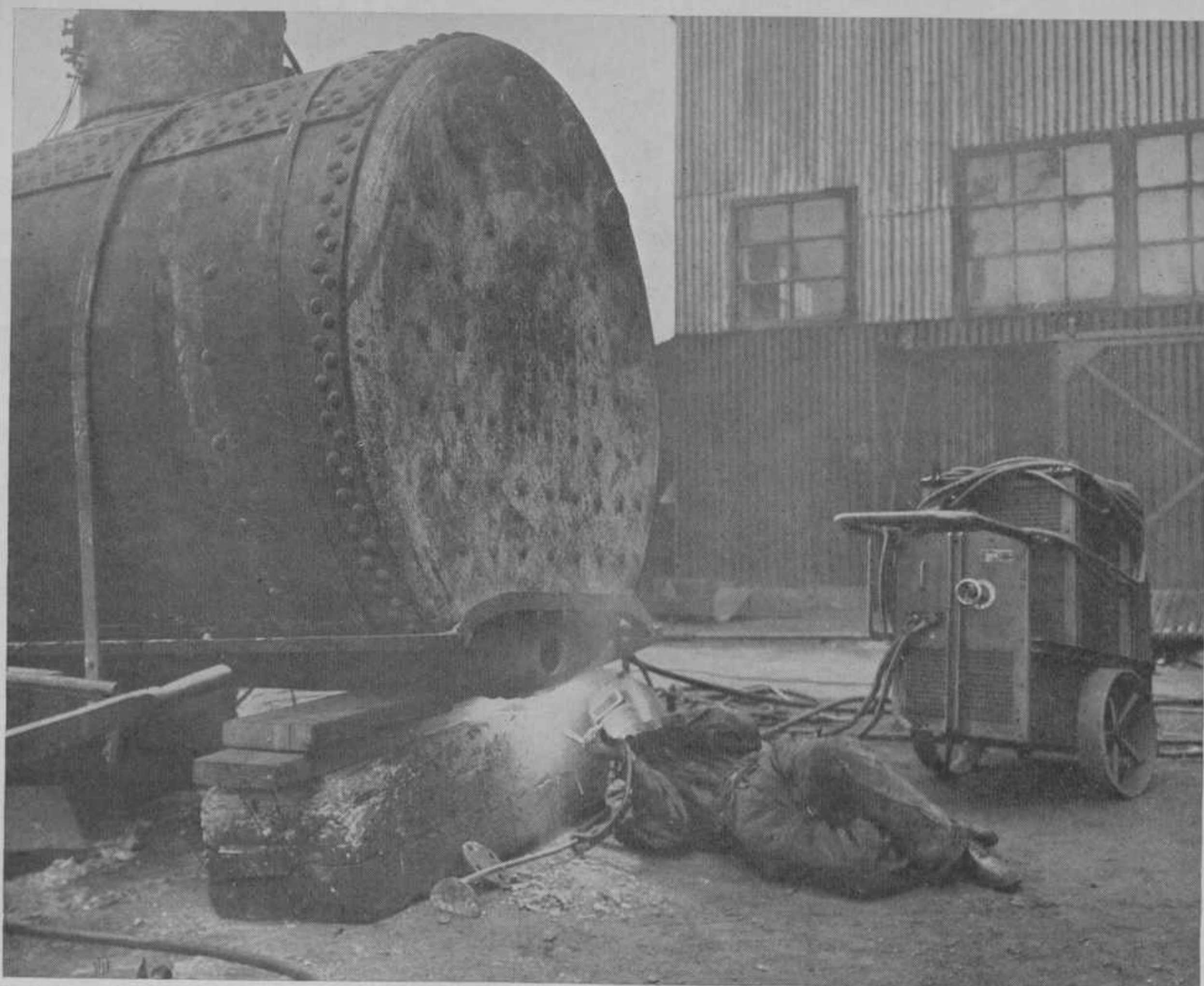
ONDEROPLOSSCHEN VAN EEN LEKKEN KLINKNAAD
