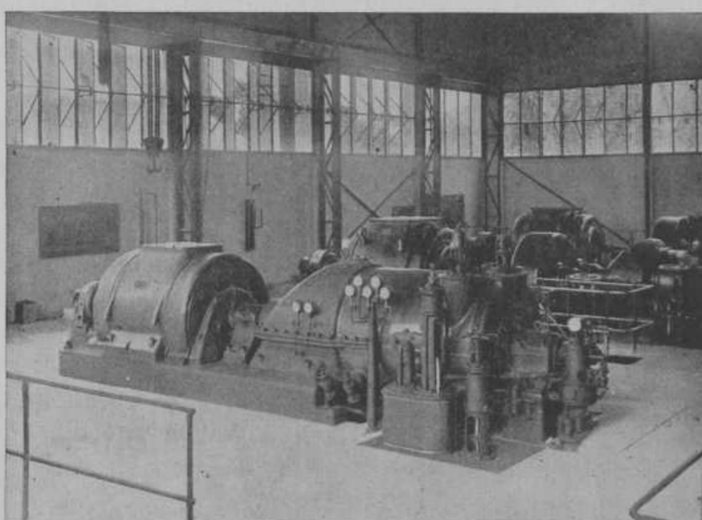
ELECTRISCHE CENTRALE PALEMBANG
