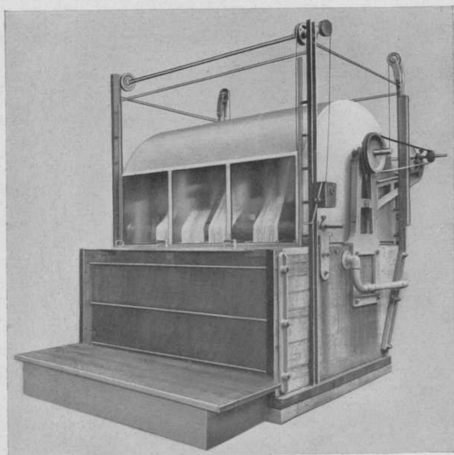
HASPELKIIP MET ROESTVRIJSTALEN BEKLEEDING EN AFNEEMBARE ROESTVRIJSTALEN BEKAPPING
