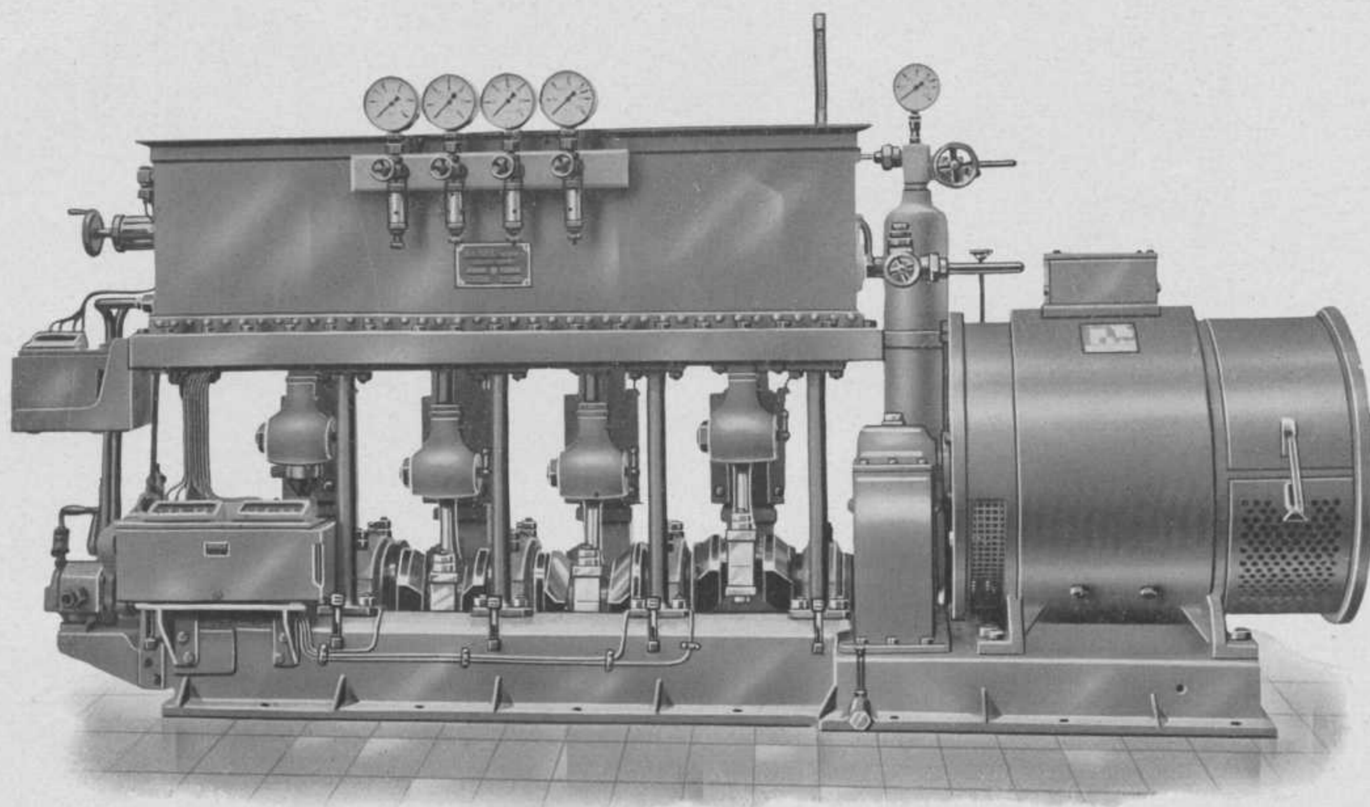
Viertredige luchtcompressor \pm 110 \text{ M}^3/\text{uur} . 225 atm., indirect gekoppeld met electomotor
