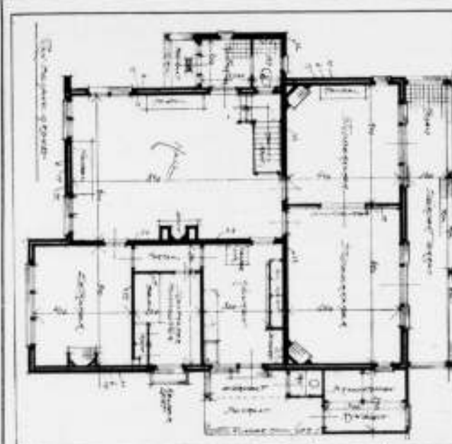
Woonhuis „de Papaver“ aan den Breede weg te Bussum. Grondplan.
