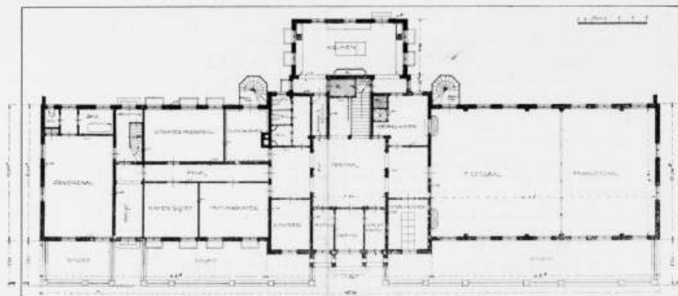
Plan van den beganen grond van het „Observatorium“.
