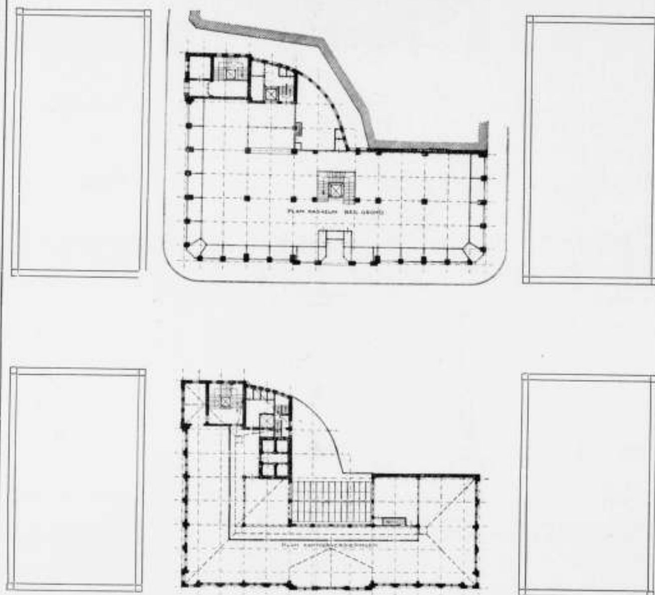
Plattengronden van het nieuwe gebouw der Firma Peck en Cloppenburg aan den Dam.
