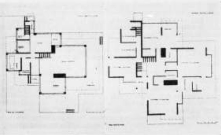
TWEE PLATTEGRONDEN VOOR EEN PARTICULIER WOONHUIS.
