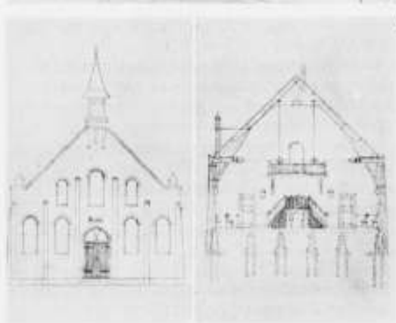
2 ONTWERP VAN EEN TIMMERMAN VOOR EEN KERKGEBOUW TE ZAA- DIJK. 1922. (Aanbesteed.)
