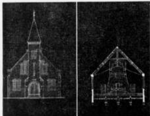
DOOR EEN AANNEMER GEWIJZIGD ONTWERP- KERKGEBOUW TE ZAA- DIJK. 1922. (Met bouwen 3 begonnen.)
