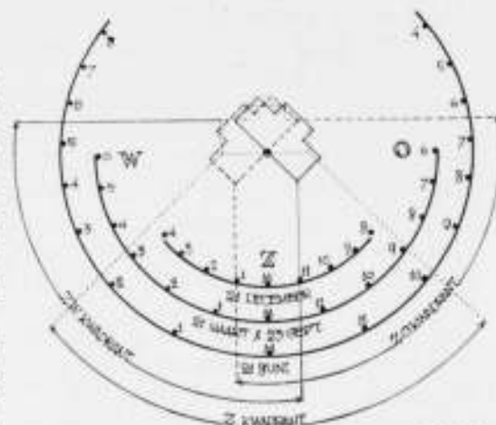
Diagram van den zonnestand op 52° N.B. (Hoek van Holland - Arnhem - Winterswijk).
