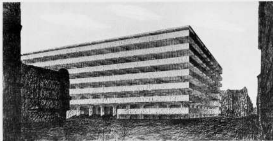
MIES VAN DER ROHE (BUROHAUS) IDEEËNPROJECT IN BETON, IJZER EN GLAS. Bij een dragende balkconstructie een nietdragende wand. De diepte van de ruimte is 16 Meter. „Ein zweistieliger Rahmen von 8 Meter Spannweite” met aan beide zijden console-overbouw van 4 Meter is het constructiebeginsel. De afstand van balk tot balk is 5 Meter. Het balksysteem draagt de vloerplaten, die aan de einden der console-armen lood boven elkaar gesteld de buitenwand vormt. Over de 2 Meter hoge buitenwand loopt een tot aan de volgende vloer reikende ononderbroken vensterreeks. Dus: zuivere „Knochen- und Hauthau”.
