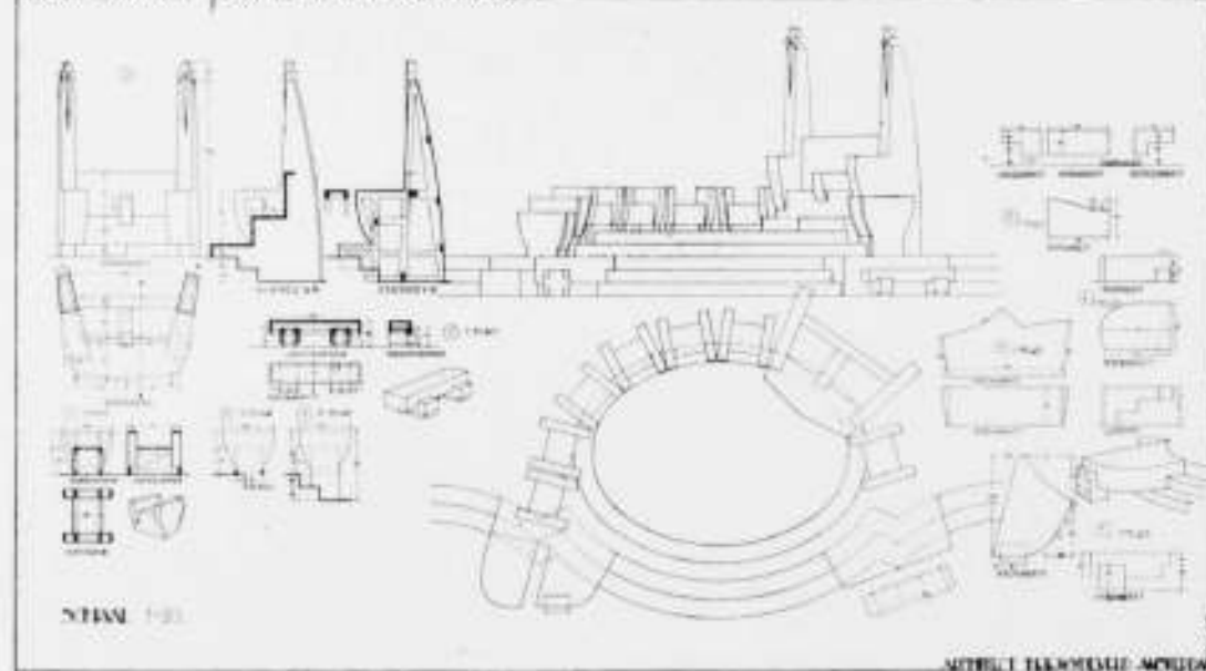
Werktekening voor decor van het zesde tafereel: DE RECHTSZITTING.
