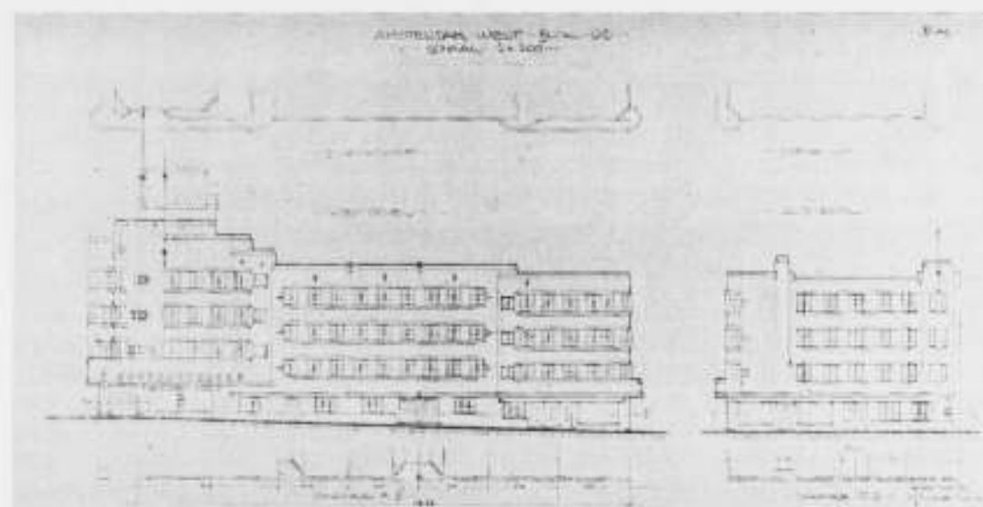
GEVELWANDEN A. D. ADMIRALENGRACHT (rechts) ARCH. J. M. VAN DER MEY
