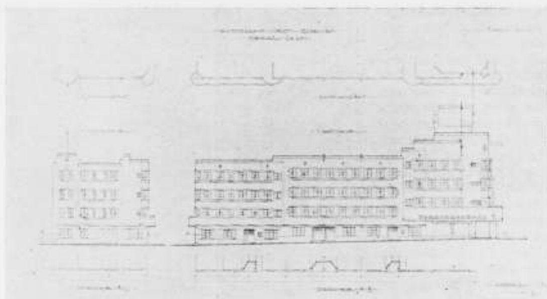
GEVELWANDEN A. D. ADMIRALENGRACHT (links) ARCH. J. M. VAN DER MEY
