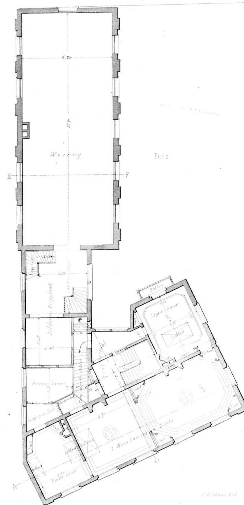
Plan van de eerste Verdieping
