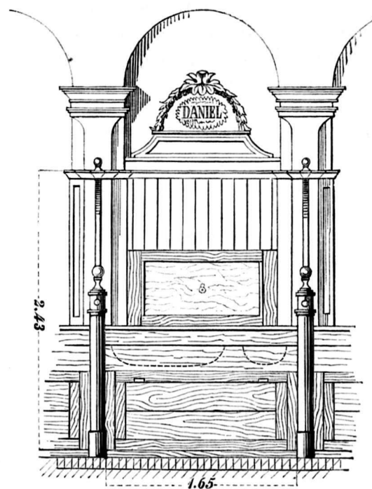
Opstand. Fig. 7.
