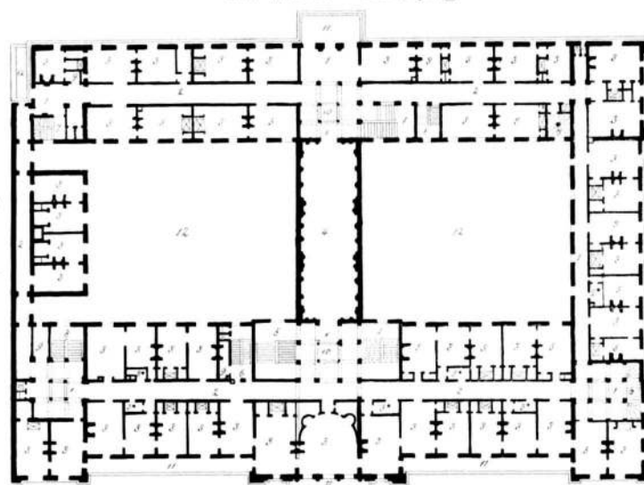
Plan van de 1 ste Verdieping
