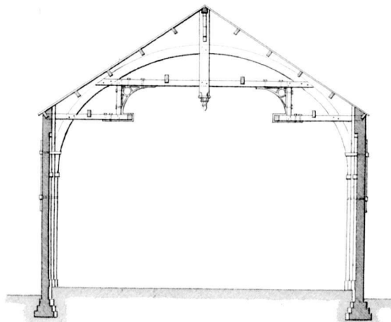
Doorsnede over de breedte
