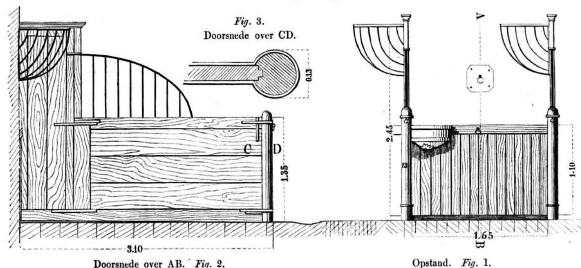
Doorsnede over AB. Fig. 2.
