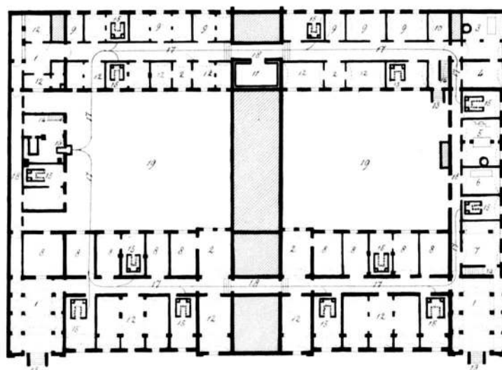
Plan van de Kelderverdieping
