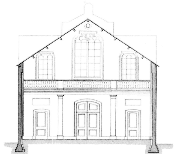
Doorsnede voor de tribune
