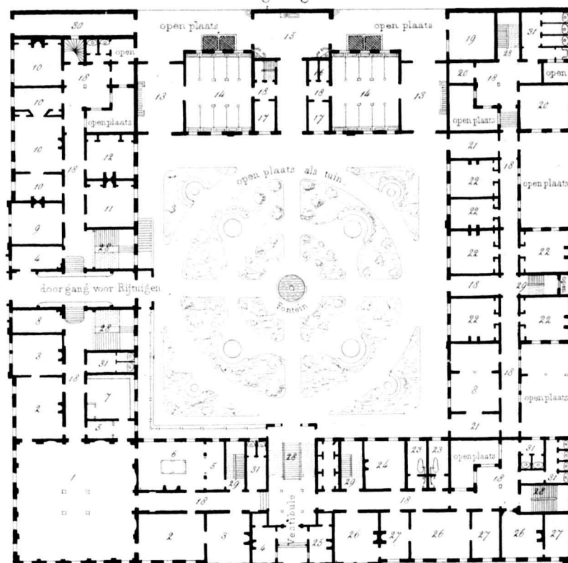
Begane grond.
