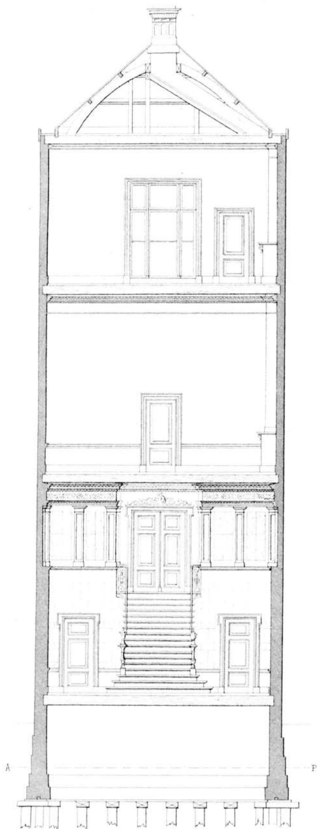
Doorsnede over AB.
