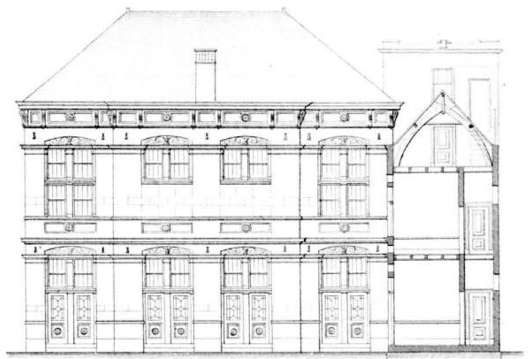
Achtergevel en Doorsnede volgens A B.
