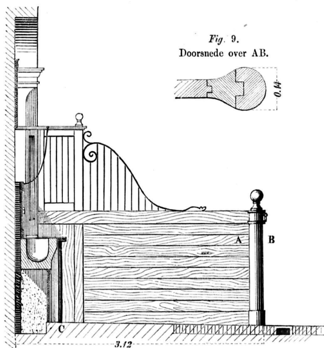
Doorsnede over de as. Fig. 8.
