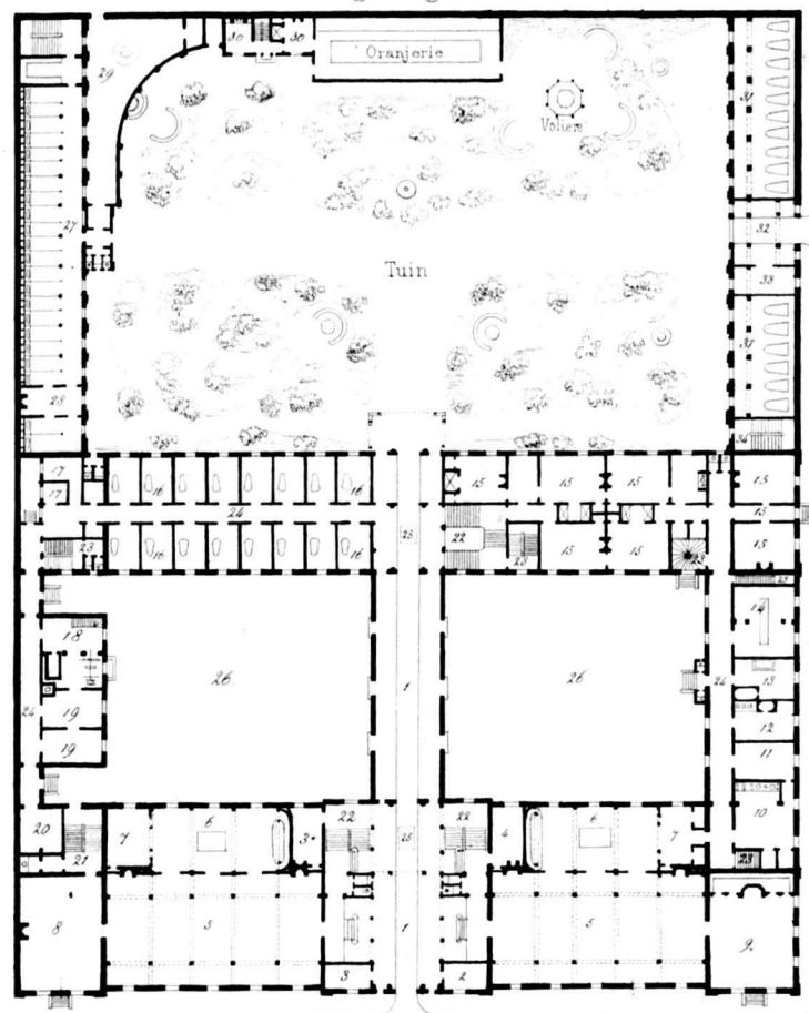
Begane grond
