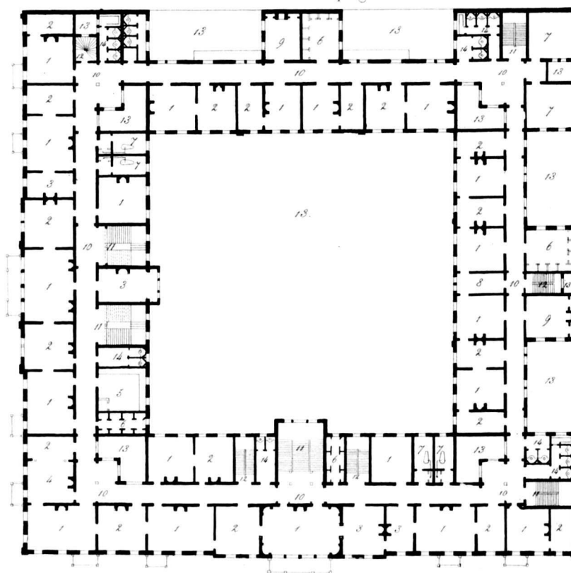
Eerste verdieping.
