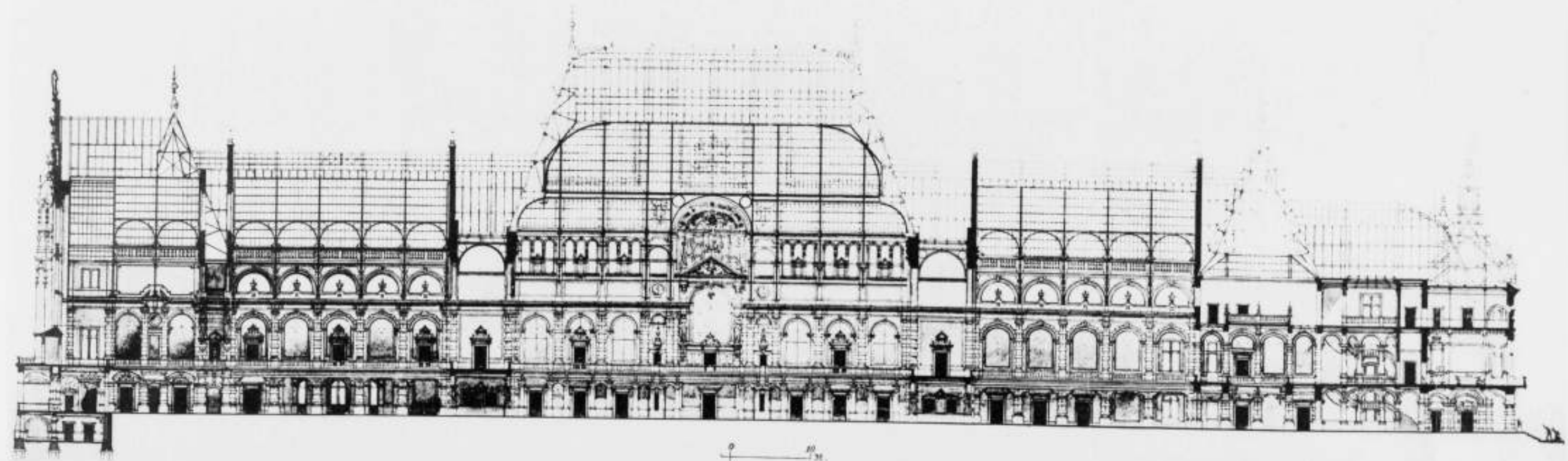
DOORSNIDE OVER DE LENGTE.
