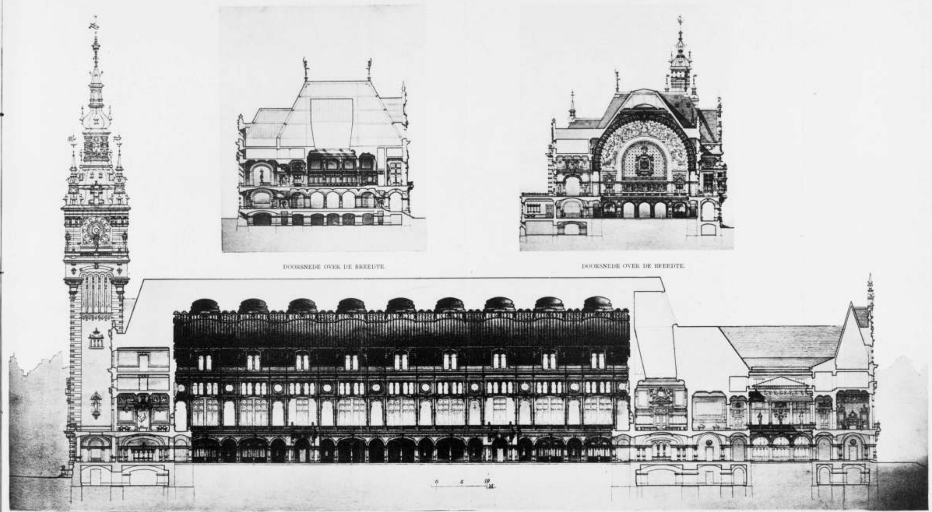
DOORSNEDE OVER DE LENGTE
