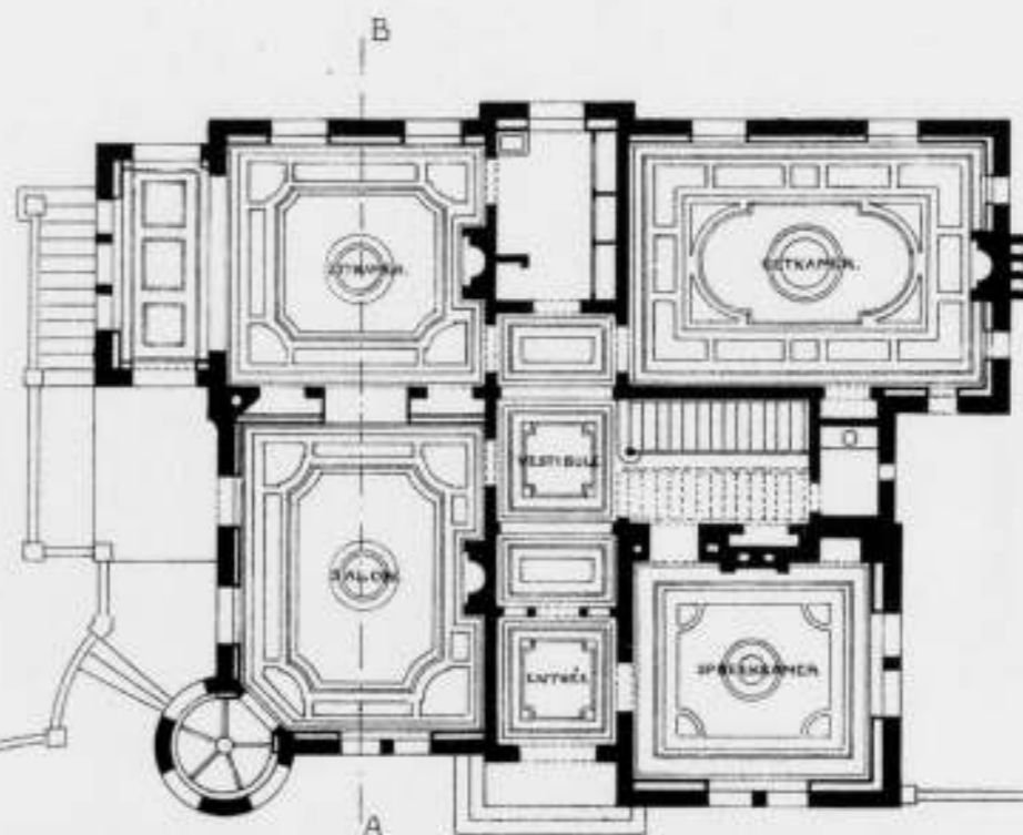
PARTERRE
