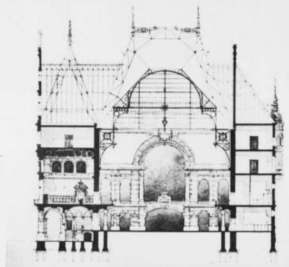
DOORSNIDE OVER DE BREEDTE.
