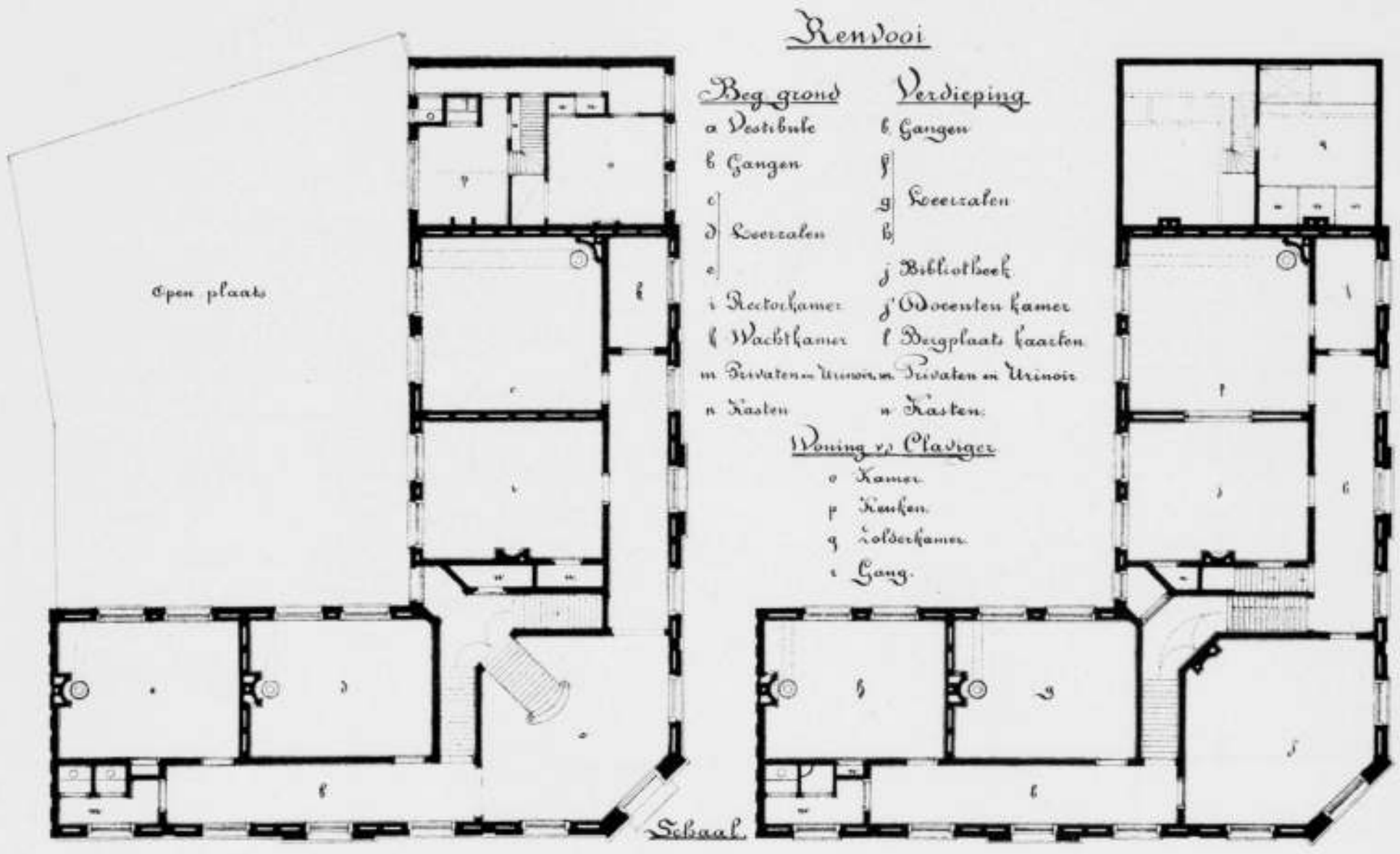
Begane grond.
