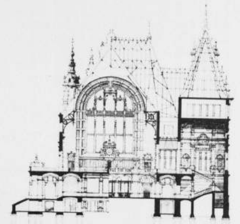
DOORSNIDE OVER DE BREEDTE.
