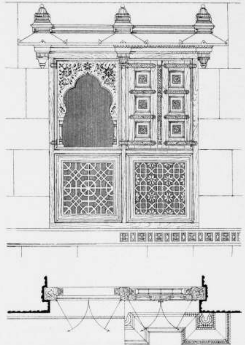
Venster van een koopmanswoning te Bombay Fenêtre d'une maison d'un négociant à Bombay
