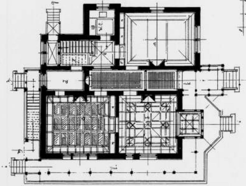
Begane Grond.
