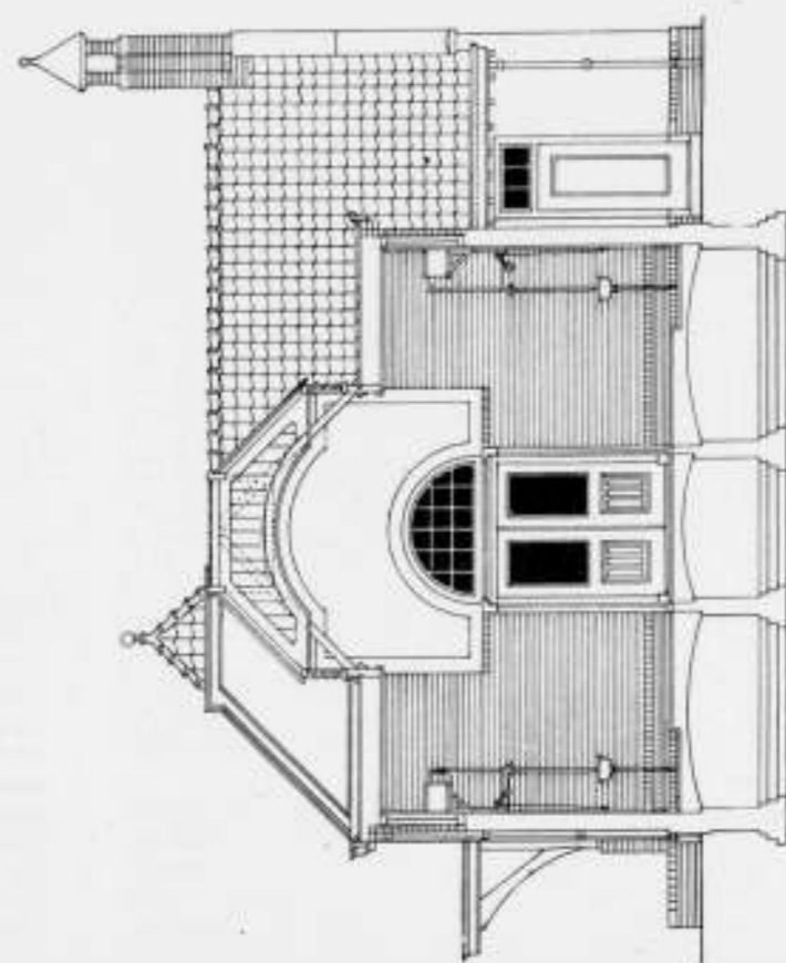
Doorsnede, Schaal 1 a 100.
