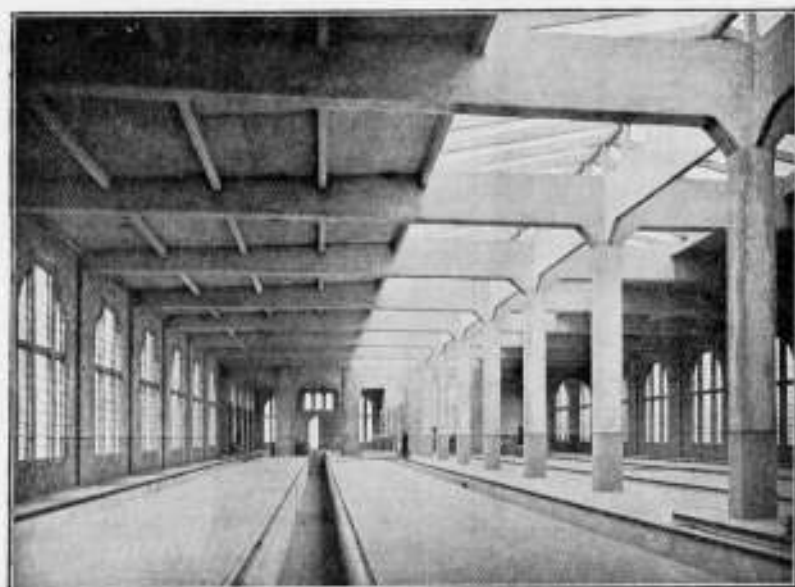
Rijtuig-remise der Z. Holl. El. Sp. Mij. te Luidschendam.
