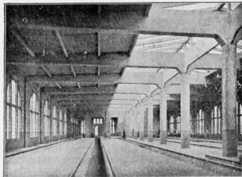
Rijtuig-waaijer der N. Holl. El. Sp. Mij. te Leidschendam.
