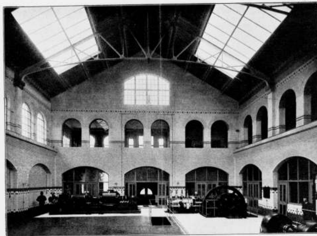
Machiniekamer.
