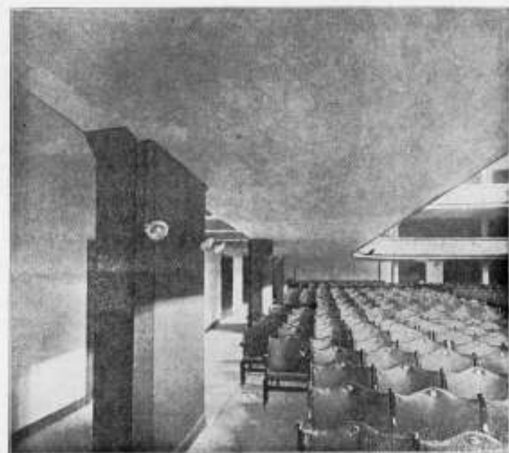
Balkon in gewapend Beton bij Geb. v. Kunsten en Wetensch. te 's-Gravenhage.
