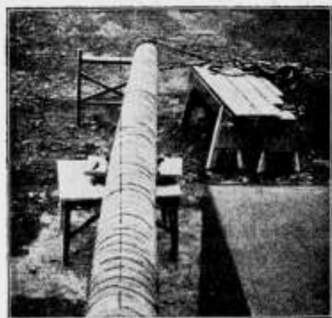
Fig. 7. Buiging van den mast tijdens de proefneming.
