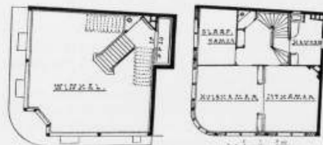
Plan beganegrond. Plan tweede verdieping. WINKELHUIS TE LEIDEN. Architecten Jesse en Fontein.
