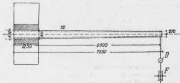
Fig. 8. Bevestigde mast voor de proefneming. D. Dynamometer. F. Katrol.
