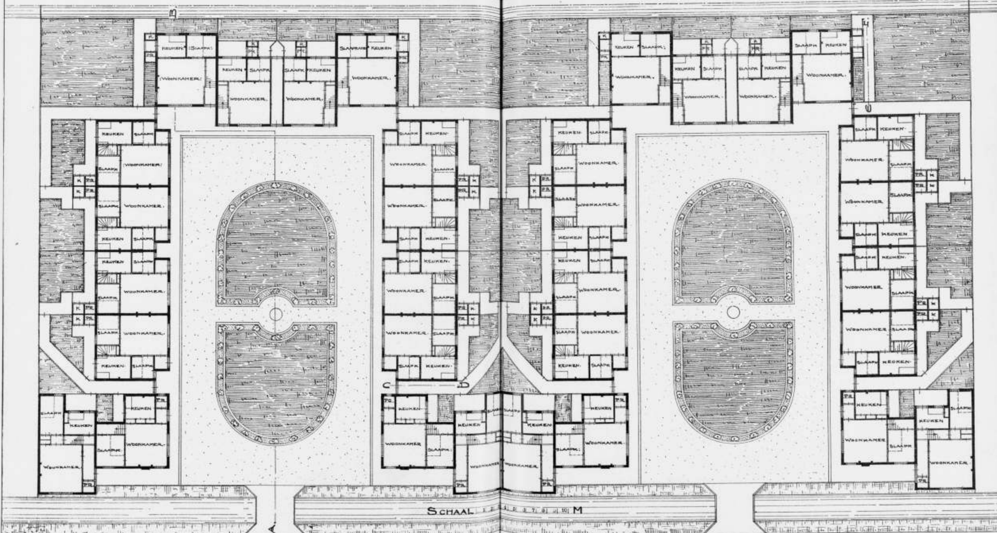
ONTWERP VOOR HET BOUWEN VAN 32 ARBEIDERSWONINGEN TE HOORN. Architect: M. J. E. Lippits, Amsterdam.
