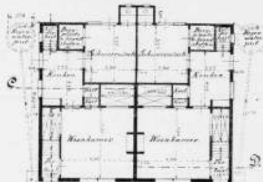
Plattegrond. „Ontwerp „Welvaart.“
