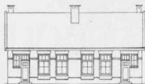
Voorgevel.
