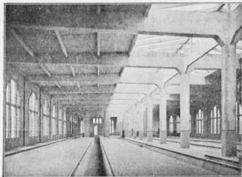
Rijtuig-remise der Z. Holl. R. Sp. Mij. te Leidschendam.
