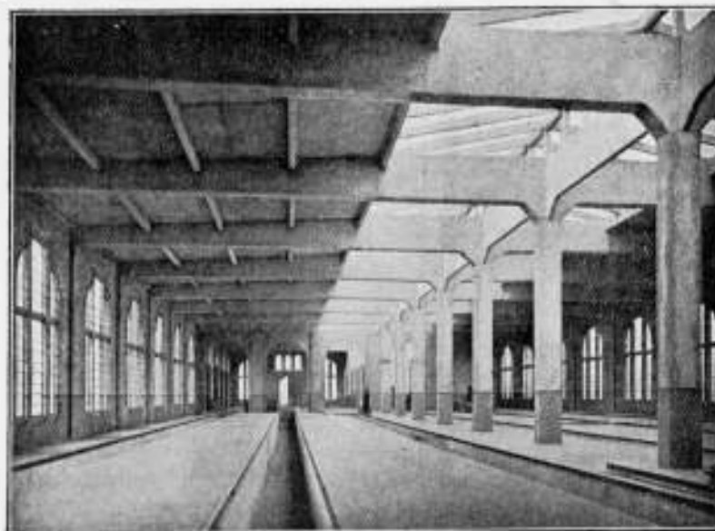
Rijtuigremise der Z. Holl. E. Sp. Mij. te Leidschendam.
