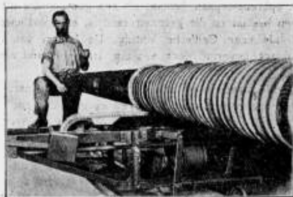
Fig. 2. Bewapenen der masten.
