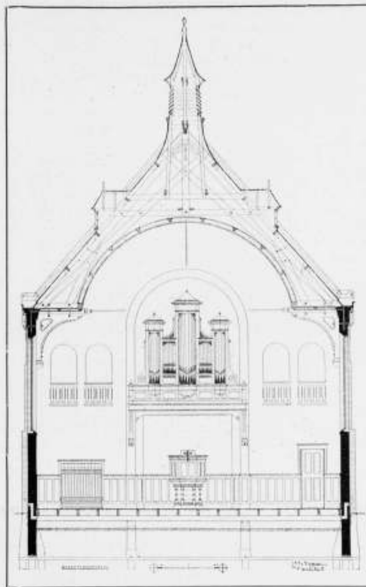
Chr. Gereform. Kerk te Haarlem.
