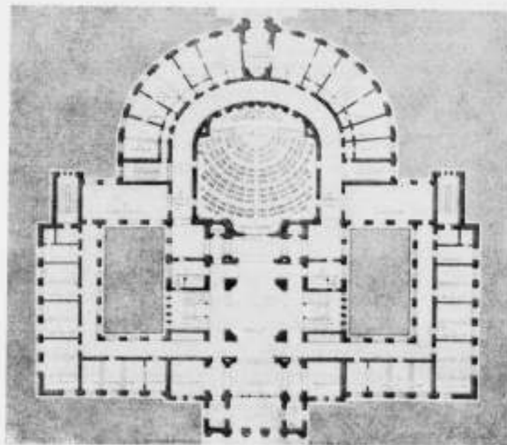
LANDDAGSGEBOUW VOOR HELSINGFORS. Plan begane grond. (Zie losse plaat). Arch. ELIEL SAARINEN.
