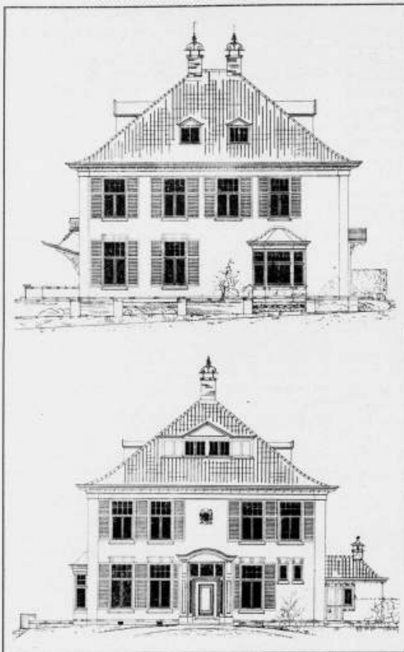
Villa „De Heerd” te Bloemendaal, Rijperweg, van den heer C. N. J. Moltzer. Voorgevel en linker zijgevel. Schaal 1 op 200. Architect Jos. Th. J. Cuypers, C. B. I. Bekroond met een zilveren medaille, uitgelooft door de gemeente Bloemendaal en door de Vereeniging: „Bloemendaal's Bloei”.
