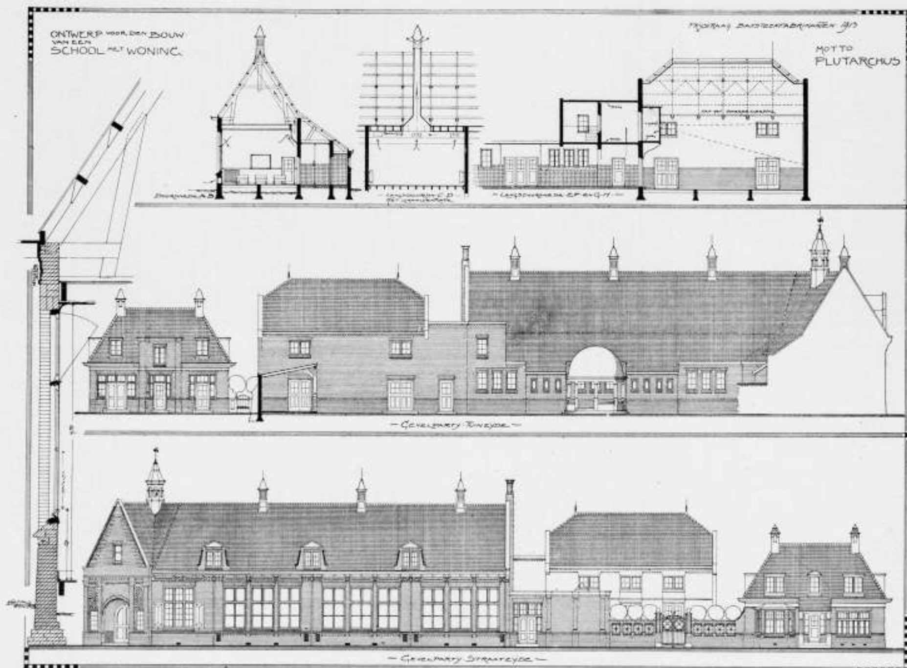
Ontwerp motto: „Plutarchus“ van PHILIPPUS J. HAMERS. GEVELS EN DOORSNEDEN. Schaal 1 op 300. DETAIL Schaal 1 op 60.
