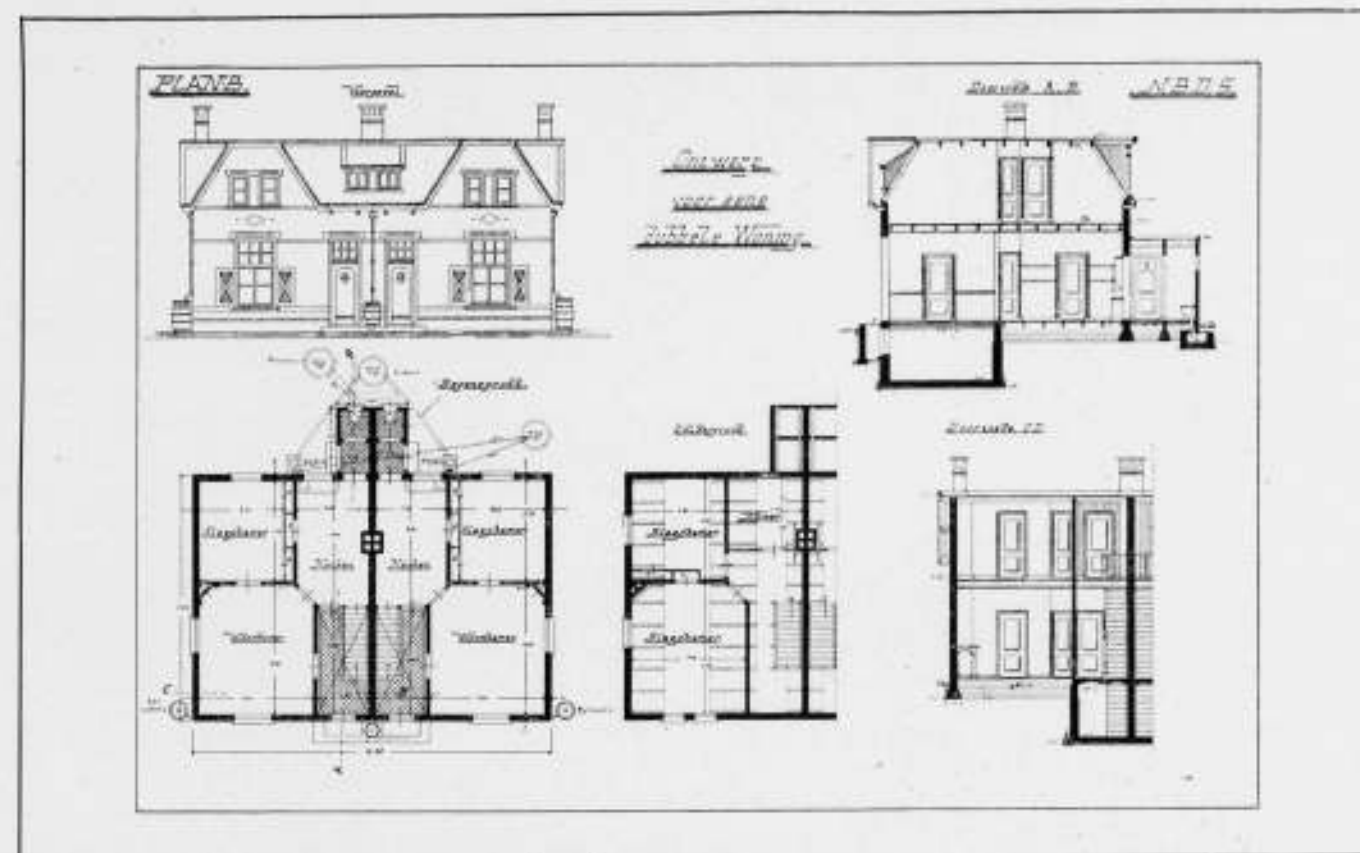
Woningtype B der N. B. D. S. te Gennep. Schaal 1 op 250.
