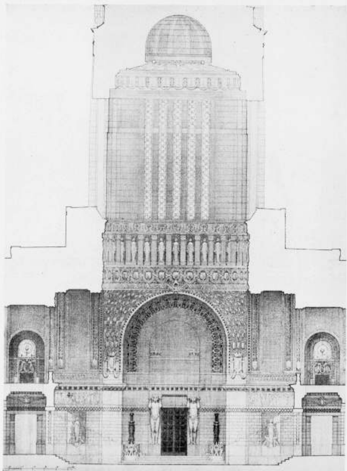
PRUJSVRAAG VREDESPALEIS. PROJECT MOTTO „L'HOMME", VAN SAARINEN. DOORSNEDE OVER DE VESTIBULE. Reproductie op \frac{1}{4} der grootte van de plaat, voorkomende in het prachtwerk „Het Vredespaleis". Zie het bericht op bladz. 462.
