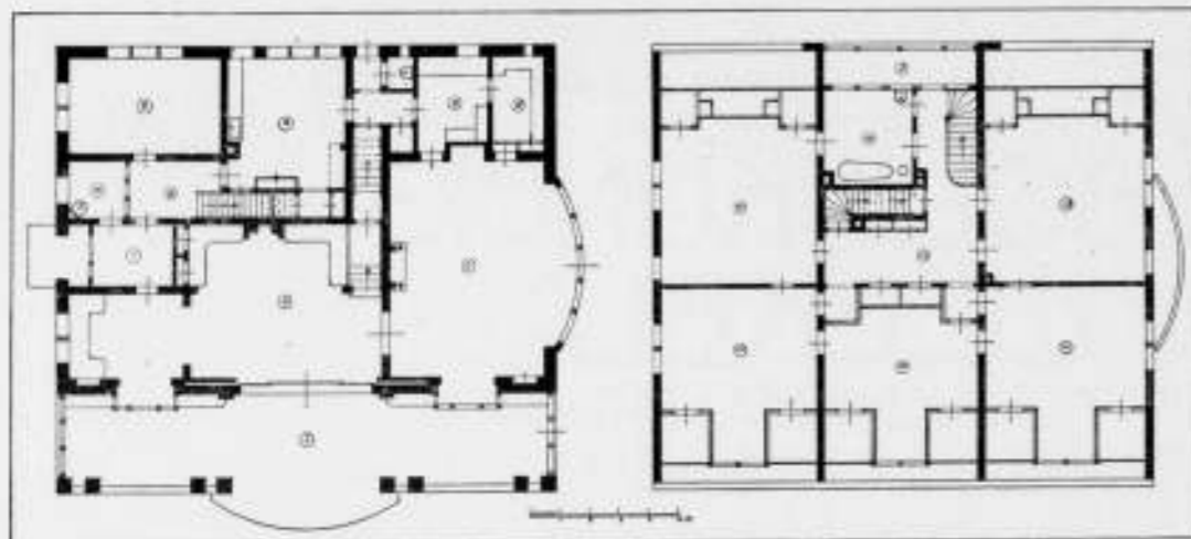
Afb. 1. Landhuis te Boekelo. Plan Begane grond en Verdieping.
