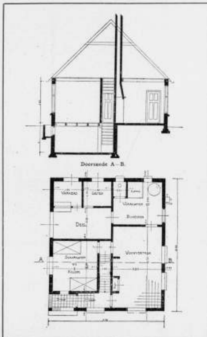
Afb. 1. Ontwerp Achterhoek B. Plattegrond en doorsnede. Ontw. G. J. Postel Hzn. Schaal 1 op 150.
