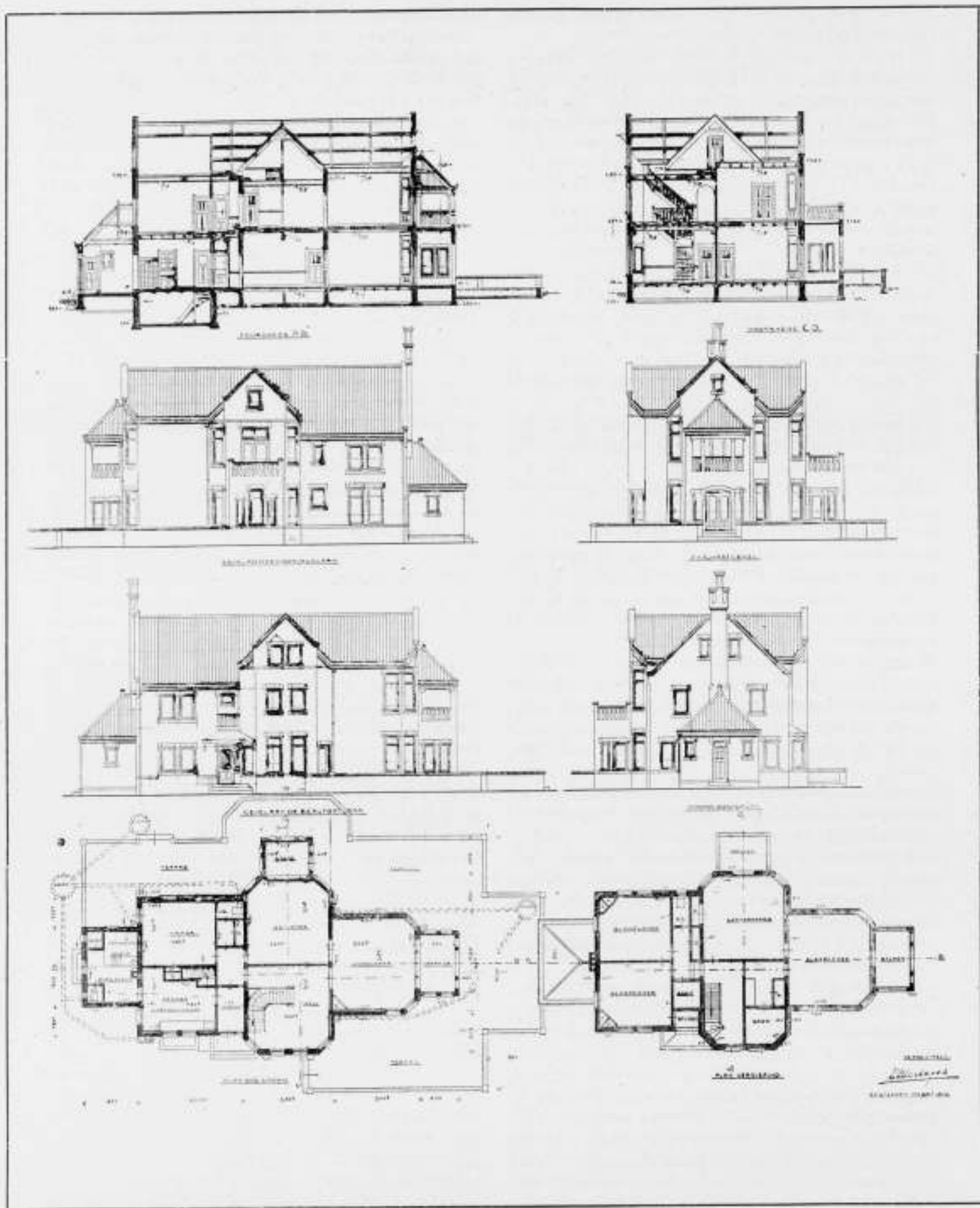
Landhuis van den Heer Dr. H. W. SALOMONSON te Baard. Plattegronden, gevels en doorsneden, Schaal 1 op 300. Arch. H. P. BERLAGE NZN.
