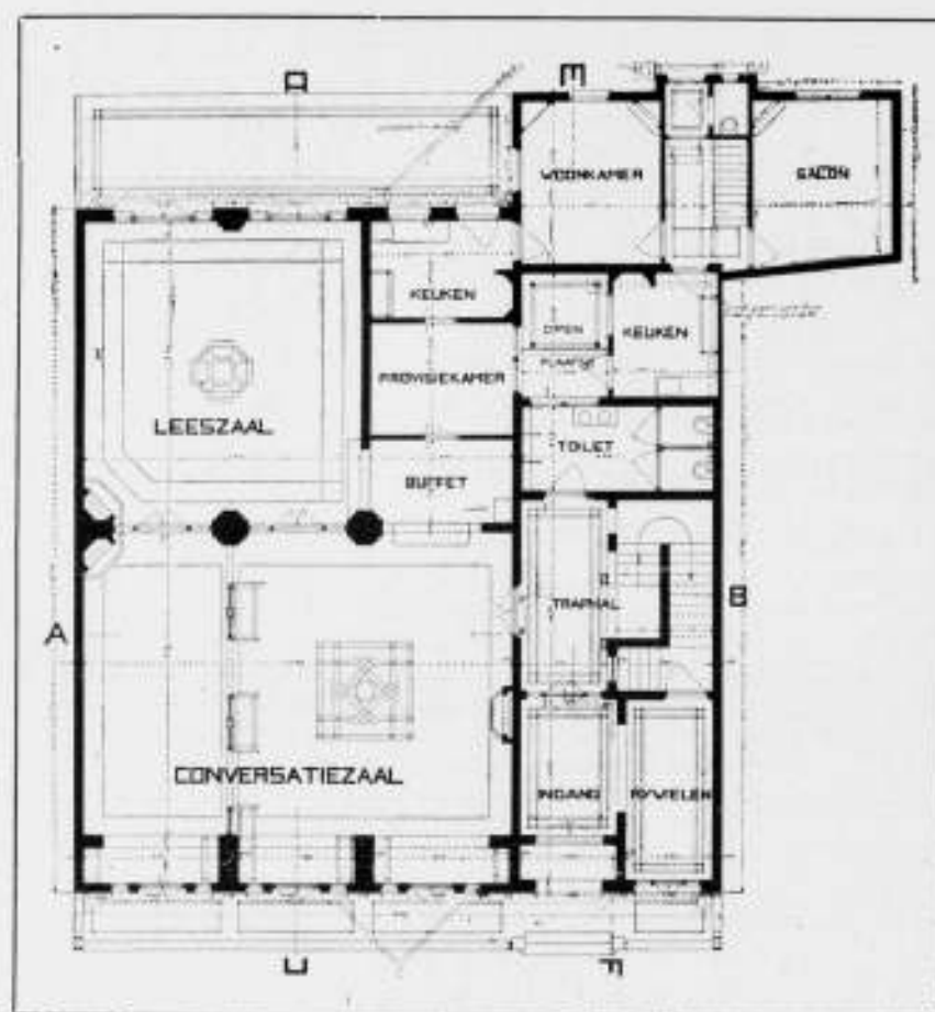
Fig. 1. Plan Beganegrond. Schaal 1 op 200.
