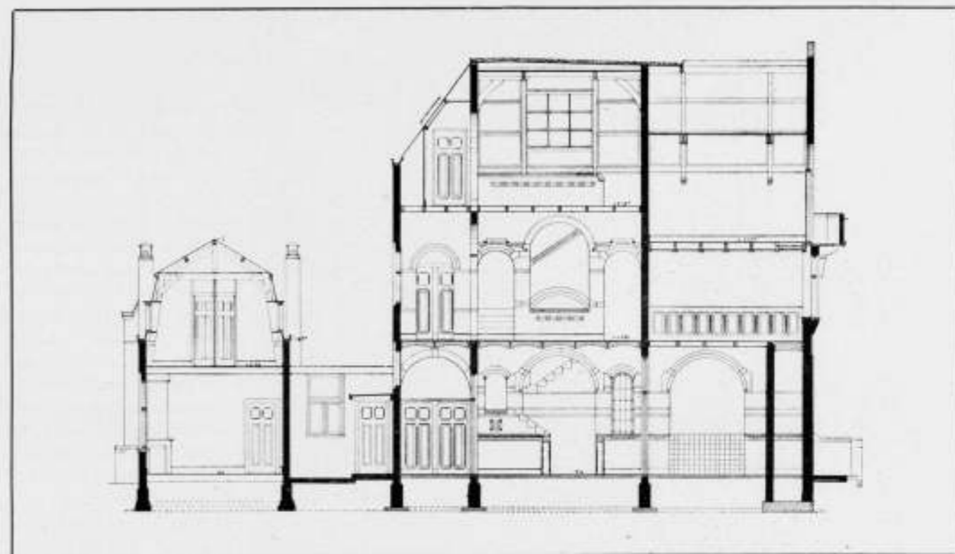
Fig. 4. Doorsnede E. F. Schaal 1 op 150.
