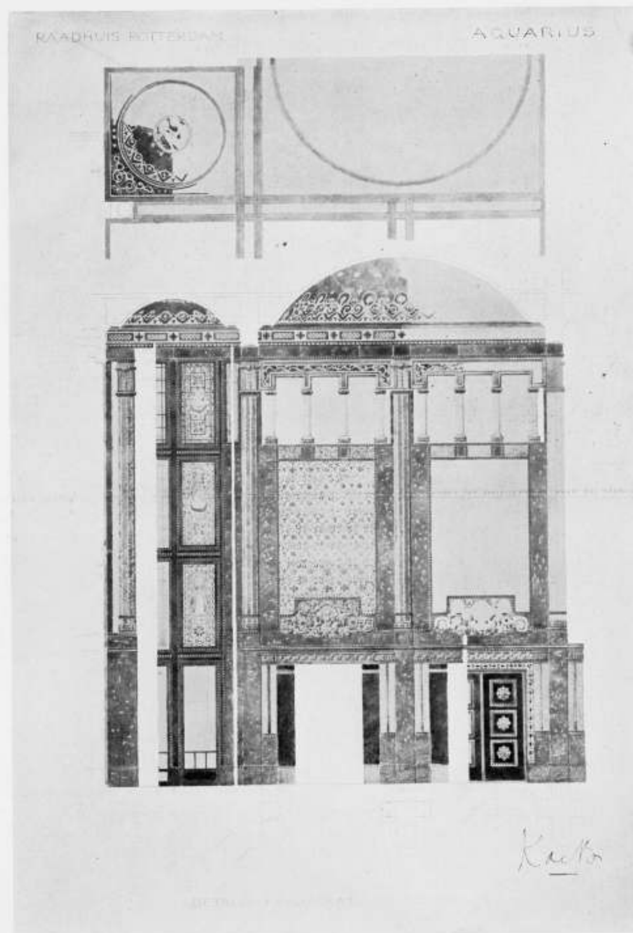
PRIJSVRAAG ROTTERDAMSCHER RAADHUIS. Ontwerp motto: AQUARIUS van K. P. C. DE BAZEL. DETAIL VAN DE FEESTZAAL.
