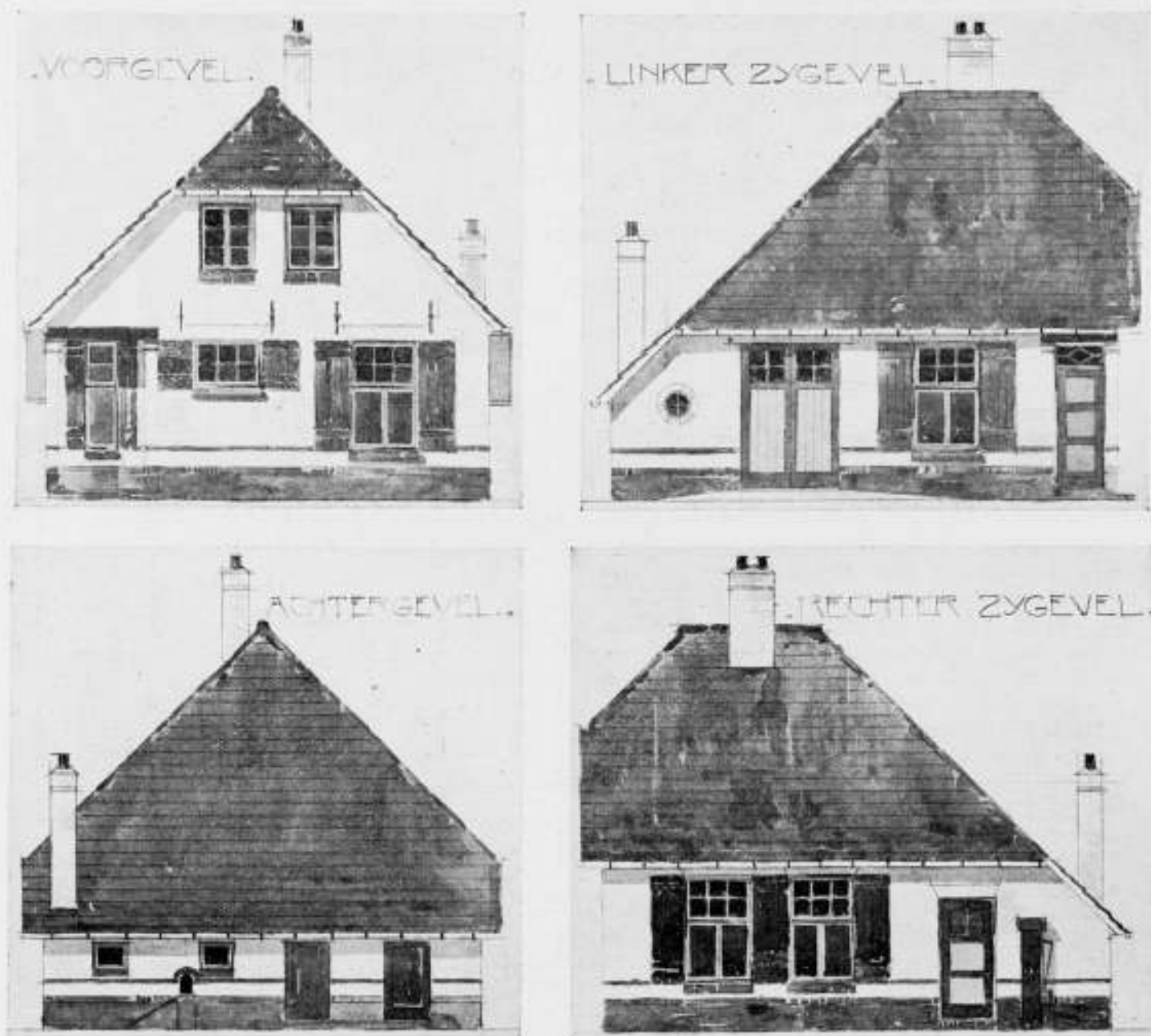
Afb. 2. Ontwerp Achterhoek B. Ontw. G. J. Postel Hzn. Schaal 1 op 100.
