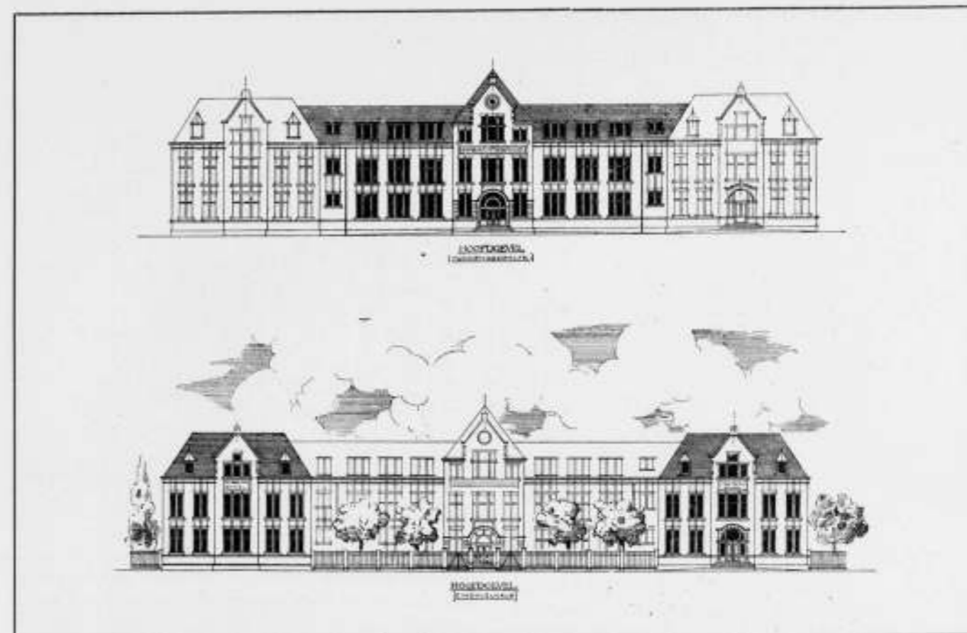
Midd. Techn. School en Ambachtsschool te Haarlem, Voorgevel. Ontwerp van P. Doorn. Ontleend aan „Schoonheid en Opvoeding“.
