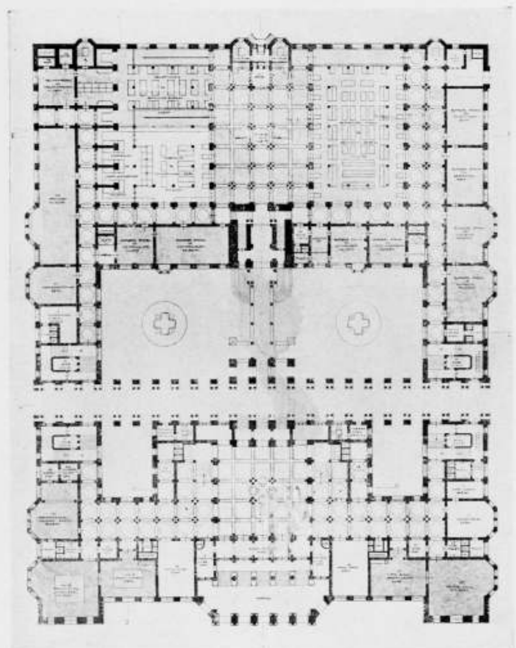
PRIJSVRAAG ROTTERDAMSCHER RAADHUIS. Ontwerp motto: „Aquarius” van K. P. C. DE BAZEL. PLAN BEGANEGROND.
