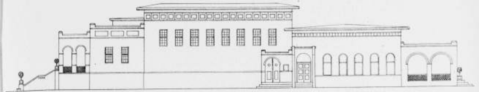
Hoofdgebouw: Theater en Restaurant. Zijgevel schaal 1 op 200
