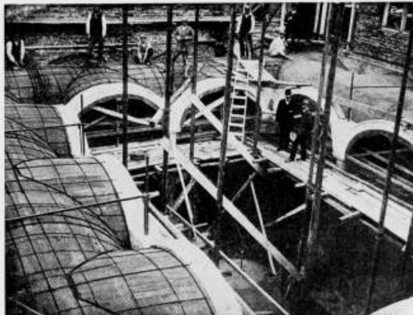
Kruisgewelven in steengas, uitgevoerd in het Bibliotheekgebouw der Technische Hoogeschool te Delft.
