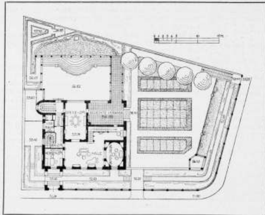
VILLA ING. AST OP DE HOHE WARTE TE WEENEN. Schaal 1 op 500. ARCH.PROF. JOSEPH HOFFMANN TE WEENEN. (Uit Moderne Banformen, Januar 1913. Verlag Julius Hoffman, Stuttgart).
