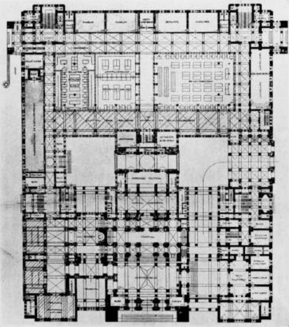
PRIJSVRAAG ROTTERDAMSCHER RAADHUIS. Ontwerp motto: „J. J.” van BRINKMAN. PLAN BEGANEGROND.
