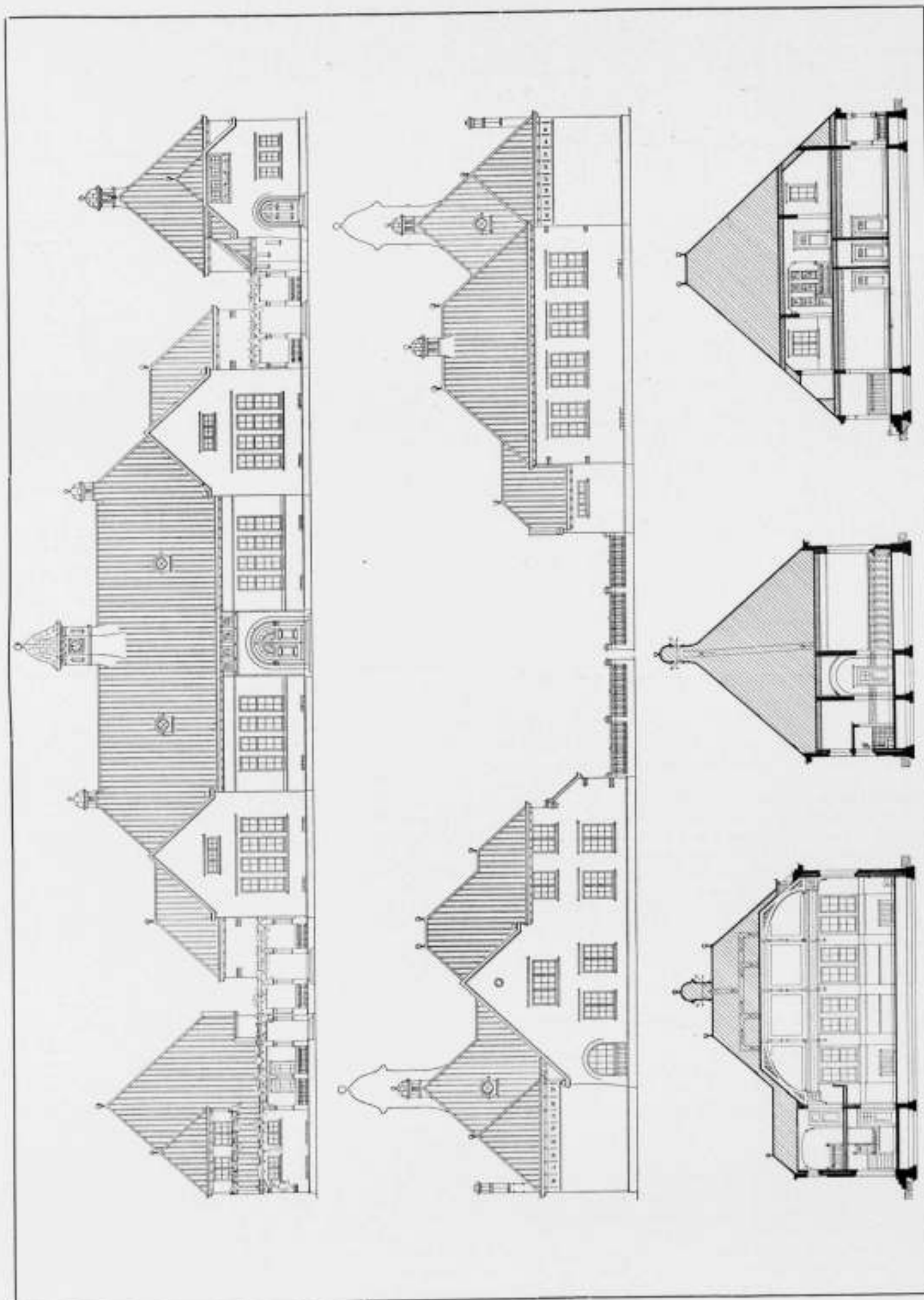
Ontwerp motto: V. M. G. van J. D. HAVERMANS, VOORGEVELS, ZIJGEVELS EN DOORSNEDEN. Schaal 1 op 300.
