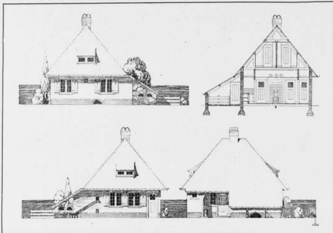
Afb. 6. Ontwerp K. N. L. V. Ontw. F. Huisbosch. Schaal 1 op 150.
