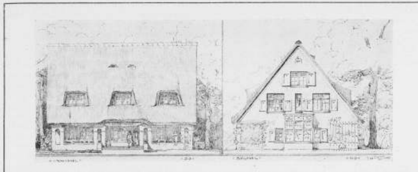
Afb. 2. LANDHUIS TE BOEKELO.
