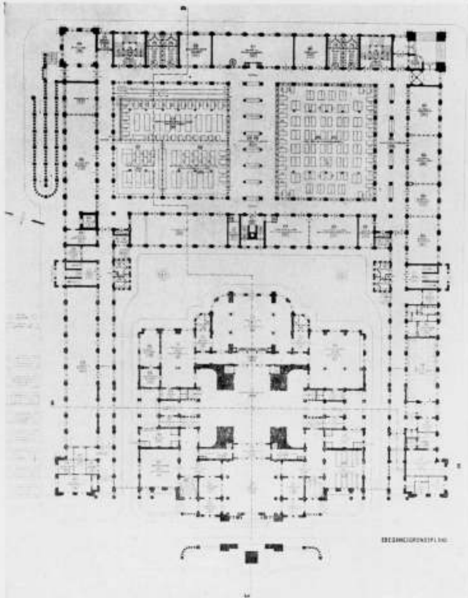
PRIJSVRAAG ROTTERDAMSCHER RAADHUIS Ontwerp motto: „Pro domo Sua” van VAN DER TAK. PLAN BEGANEGROND.
