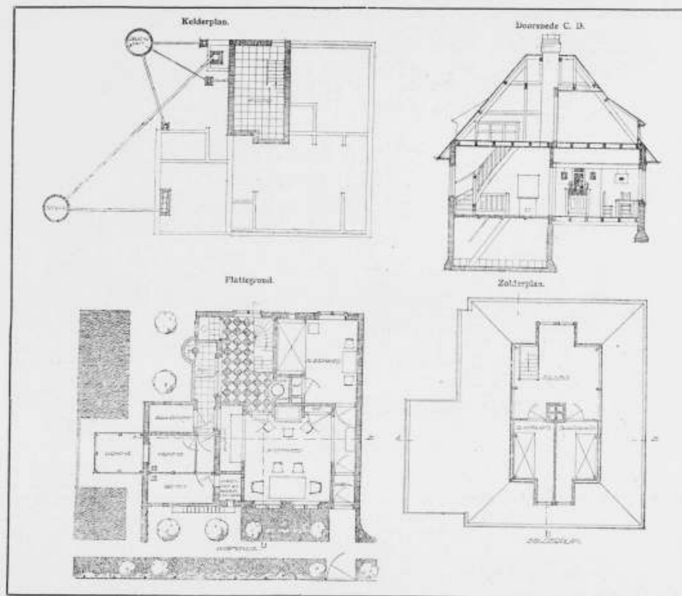
Afb. 5. Ontwerp K. N. L. V. Ontw. F. Hulsbosch. Schaal 1 op 150.
