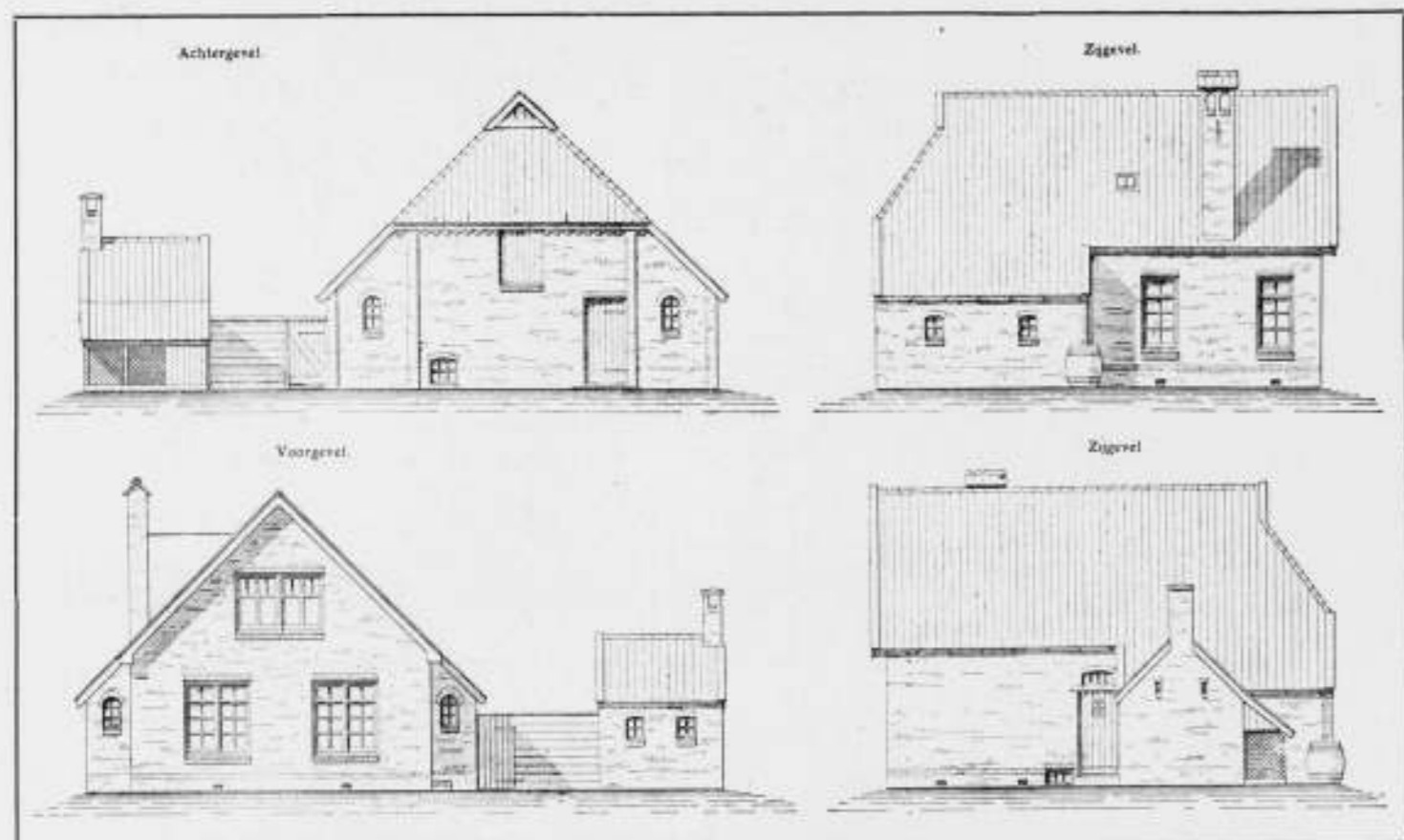
Afb. 4. Ontwerp Sub Sperati. Ontw. R. Hoff. Schaal 3 op 500.
