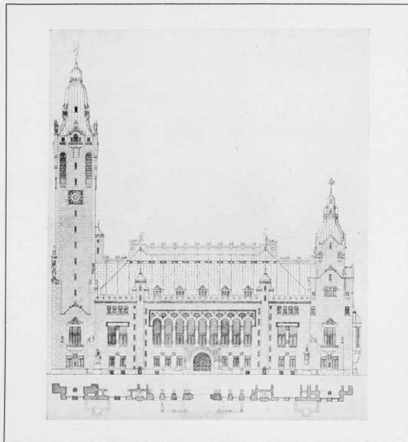
PRIJSVRAAG ROTTERDAMSCH RAADHUIS. Ontwerp: ROTERODAMI PROSPERITAS, van ALB. OTTEN en W. F. OVERIJNDER. VOORGEVEL, Schaal 1 op 600.
