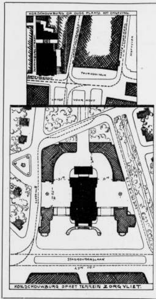
SCHETS B. Vergelijking der terreinen op dezelfde schaal, voor een Schouwburg op de bestaande plaats en op het terrein „Zorgvliet” door JOH. D. LOOYEN, Architect.
