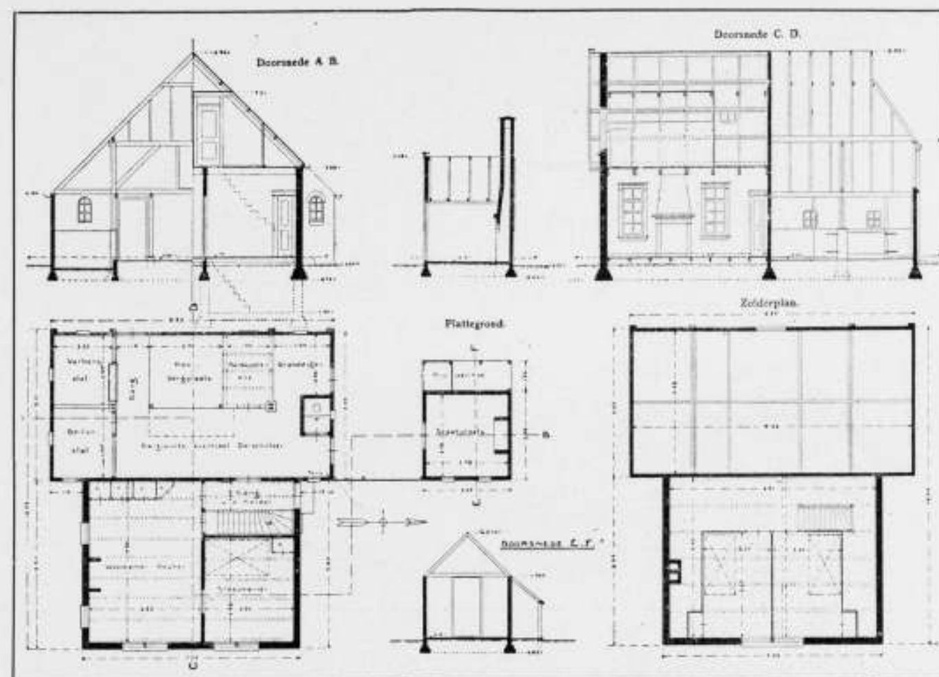
Afb. 3. Ontwerp Sub Sperati. Ontw. R. Hoff. Schaal 3 op 500.
