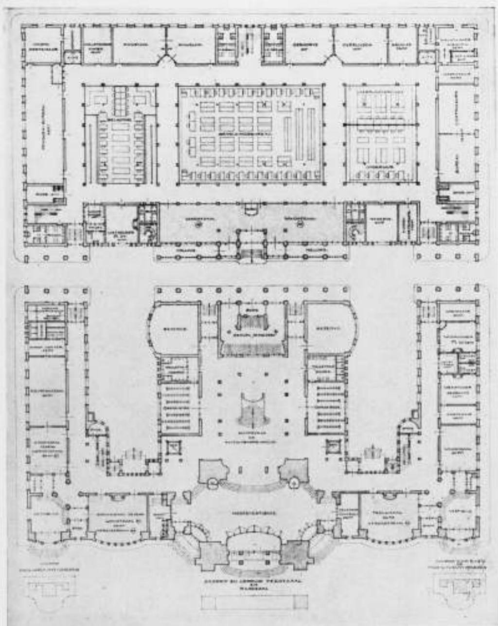
PRUISVRAAG ROTTERDAMSCHER RAADHUIS. Ontwerp motto: Representatief van W. KROMHOUT CZN. PLAN BEGANEGROND.
