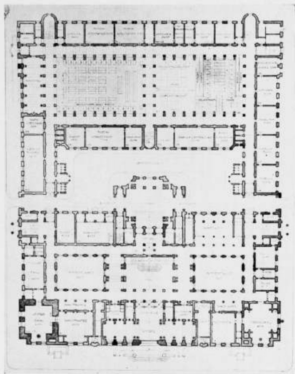
PRUISVRAAG ROTTERDAMSCHER RAADHUIS. Ontwerp motto: „Roterodami Prosperitas“ van ALB. OTTEN en W. F. OVEREIJNDER. PLAN BEGANEGROND.
