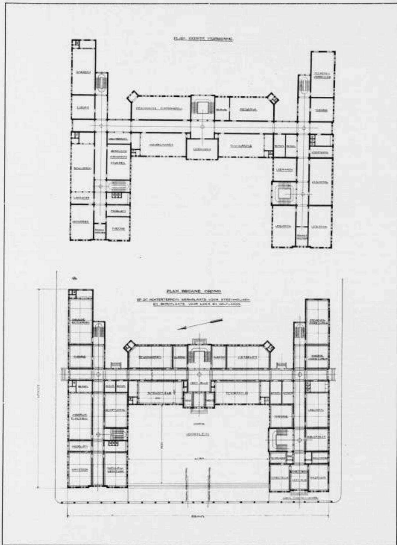
Midd. Techn. School en Ambachtsschool te Haarlem, Plan Begane grond en Eerste verdieping. Ontwerp van P. Doorn. Ontleend aan „Schoonheid en Opvoeding“.
