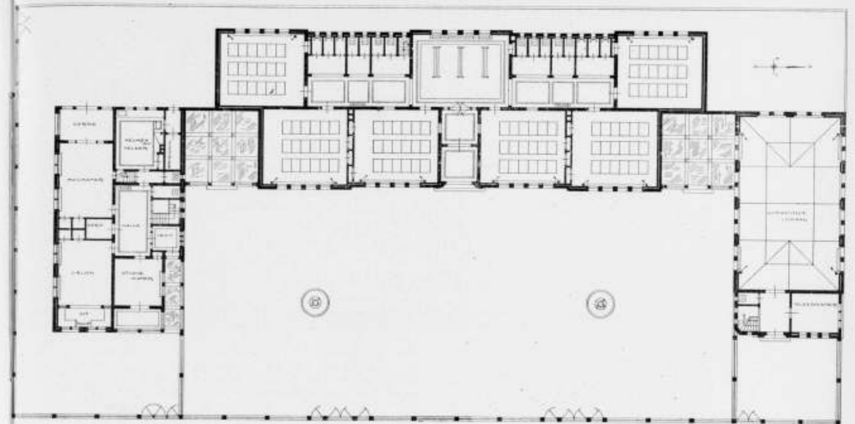
Ontwerp motto: V. M. G. van J. D. HAVERMANS — PLATTEGROND. Schaal 1 op 300.
