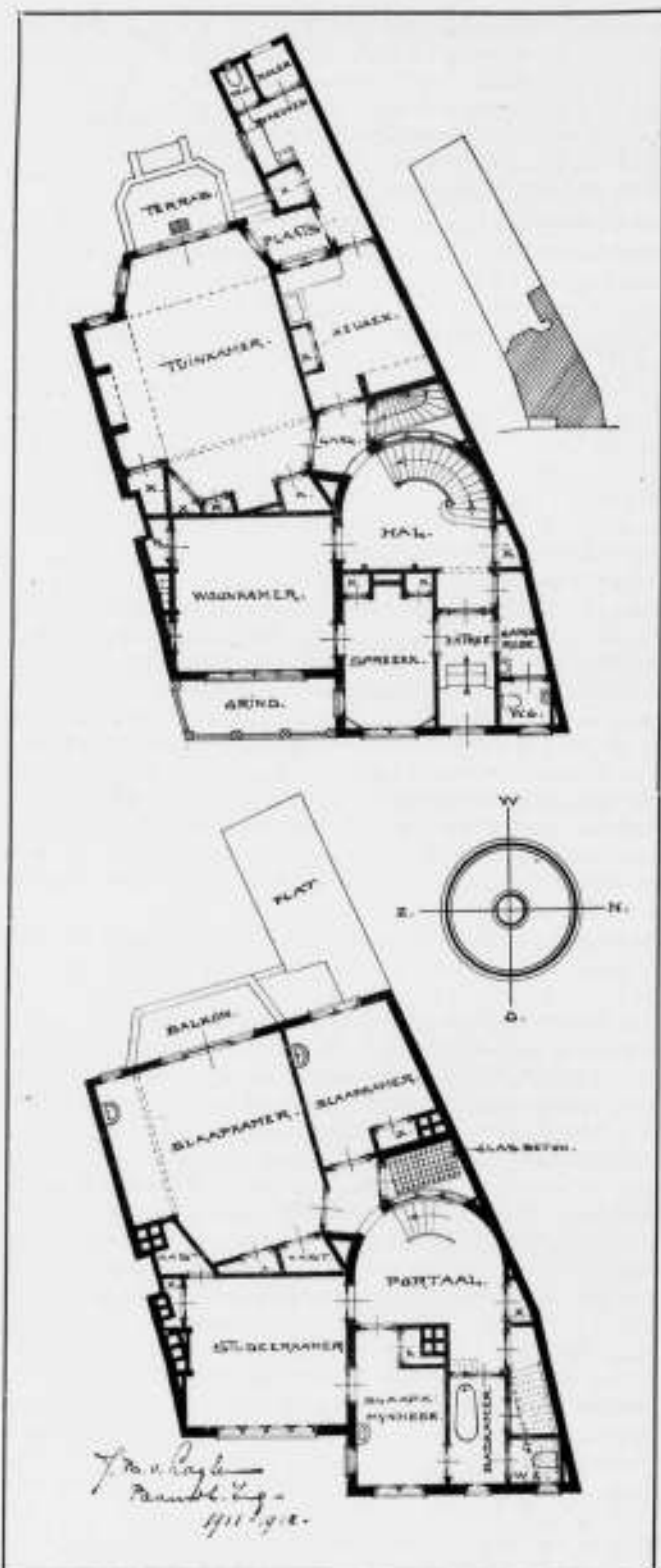
WOONHUIS TE HAARLEM. Plan Beganegrond en Verdieping. Schaal 1 op 200. Arch. J. B. VAN LOGHEM, B. I.
