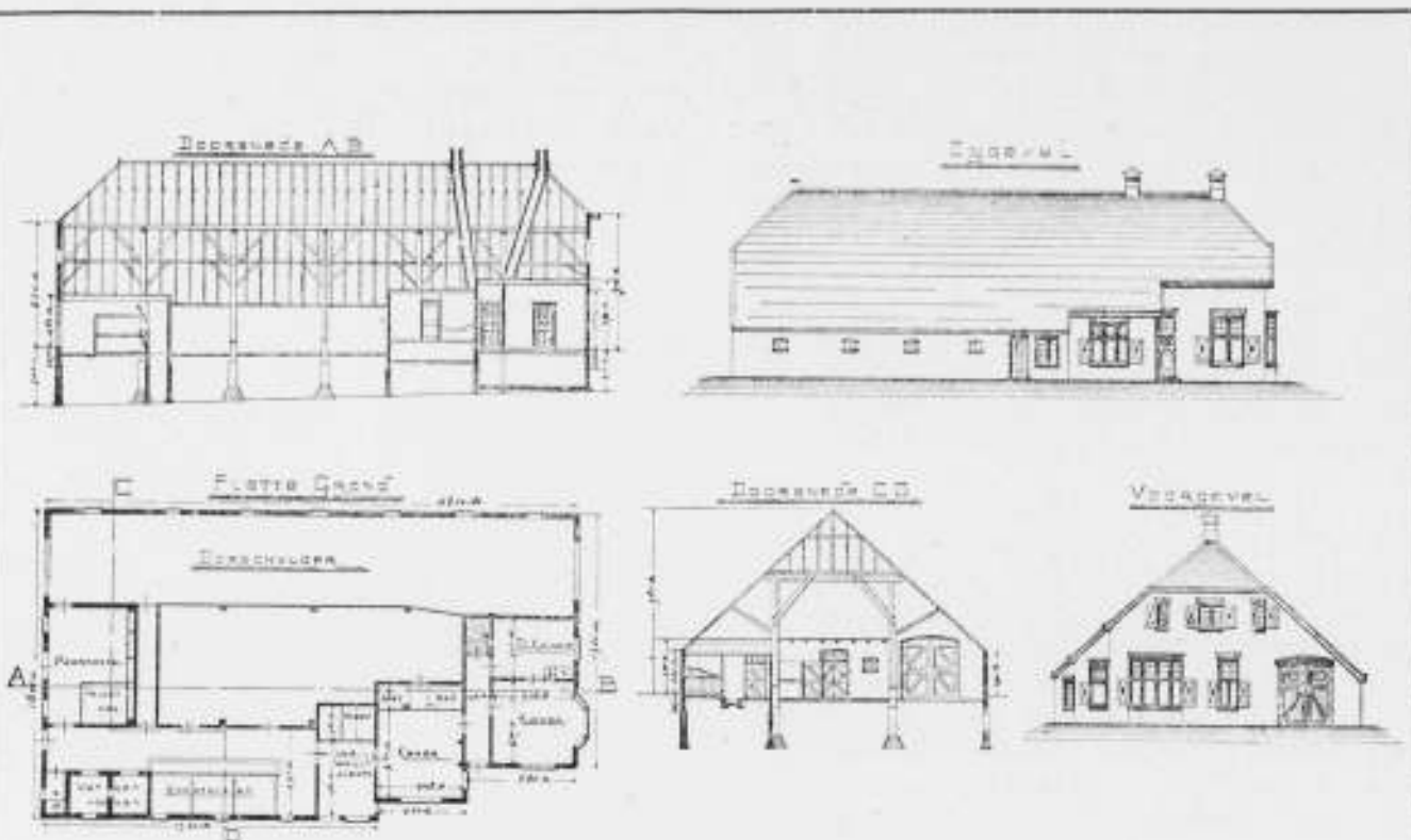
Afb. 8. Ontwerp voor een boerderij te 2de Exloërmond. Arch. A. H. Kleinberg.
