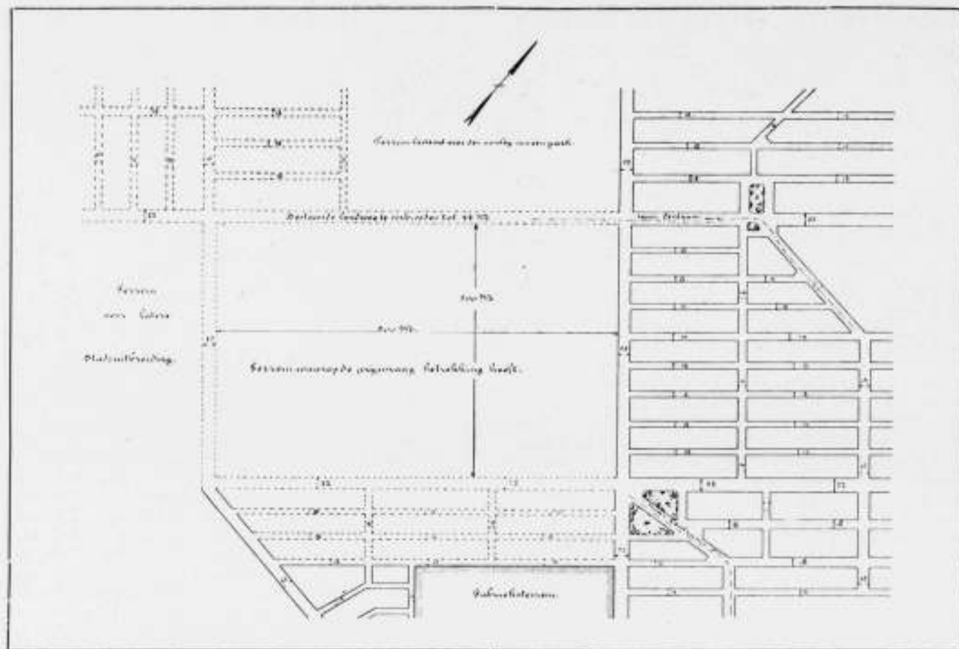
SITUATIE. SCHAAL 1 OP 10000. De bestaande straten zijn aangegeven in getrokken lijnen. De ontworpen, nog niet uitgevoerde straten, zijn aangegeven in gestippelde lijnen. De ingeschreven getallen zijn de straatbreedten in Meters. — — — — — Trambaan.
