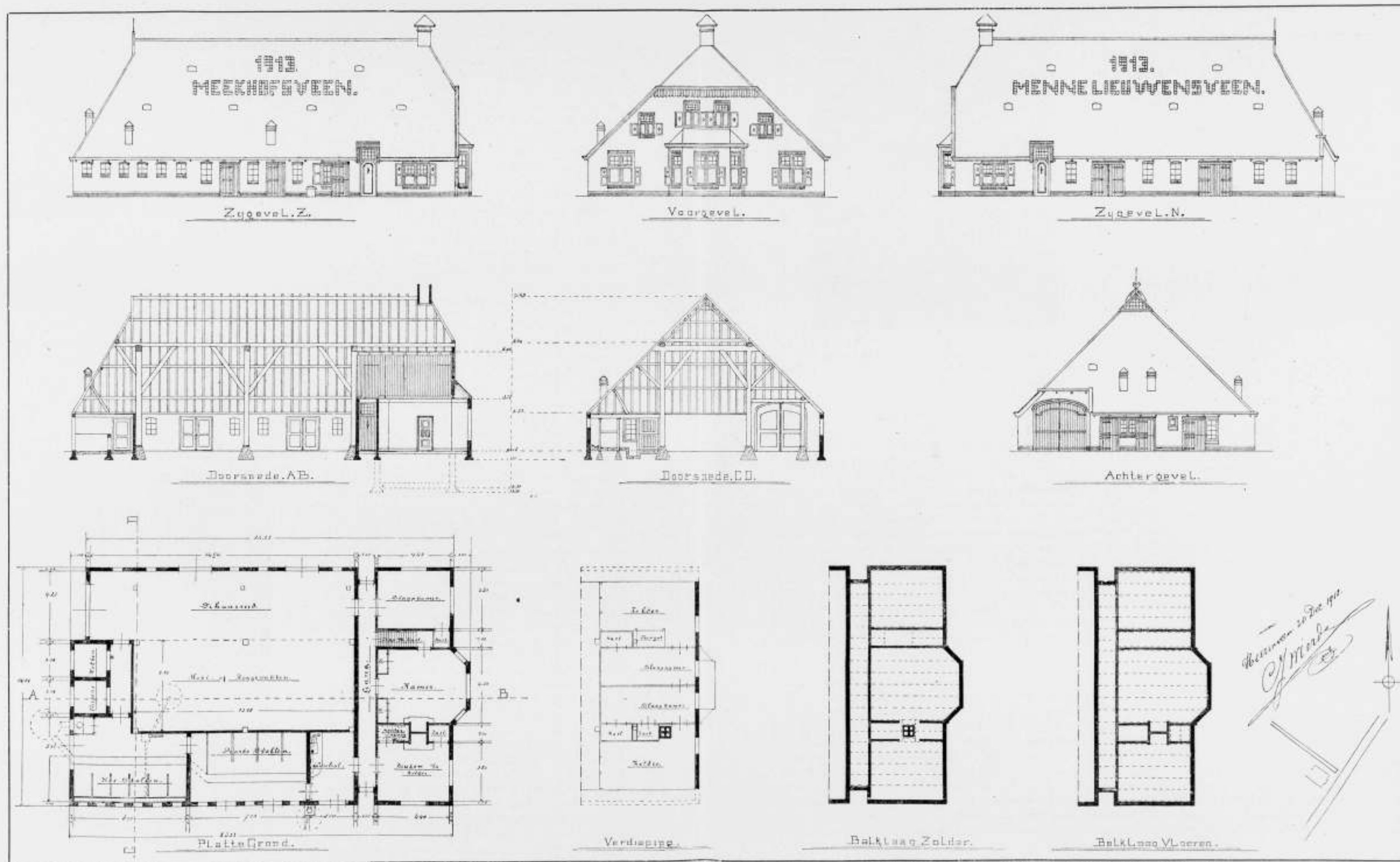
DE PRIJSVRAAG VOOR BOERDERIJEN, UITGESCHREVEN DOOR DE KON. NED. LANDBOUWVEREENIGING. Afb. 7. BOERDERIJ TE APPELSCHA, ARCHITECT C. J. WIERDA TE HEERENVEEN.
