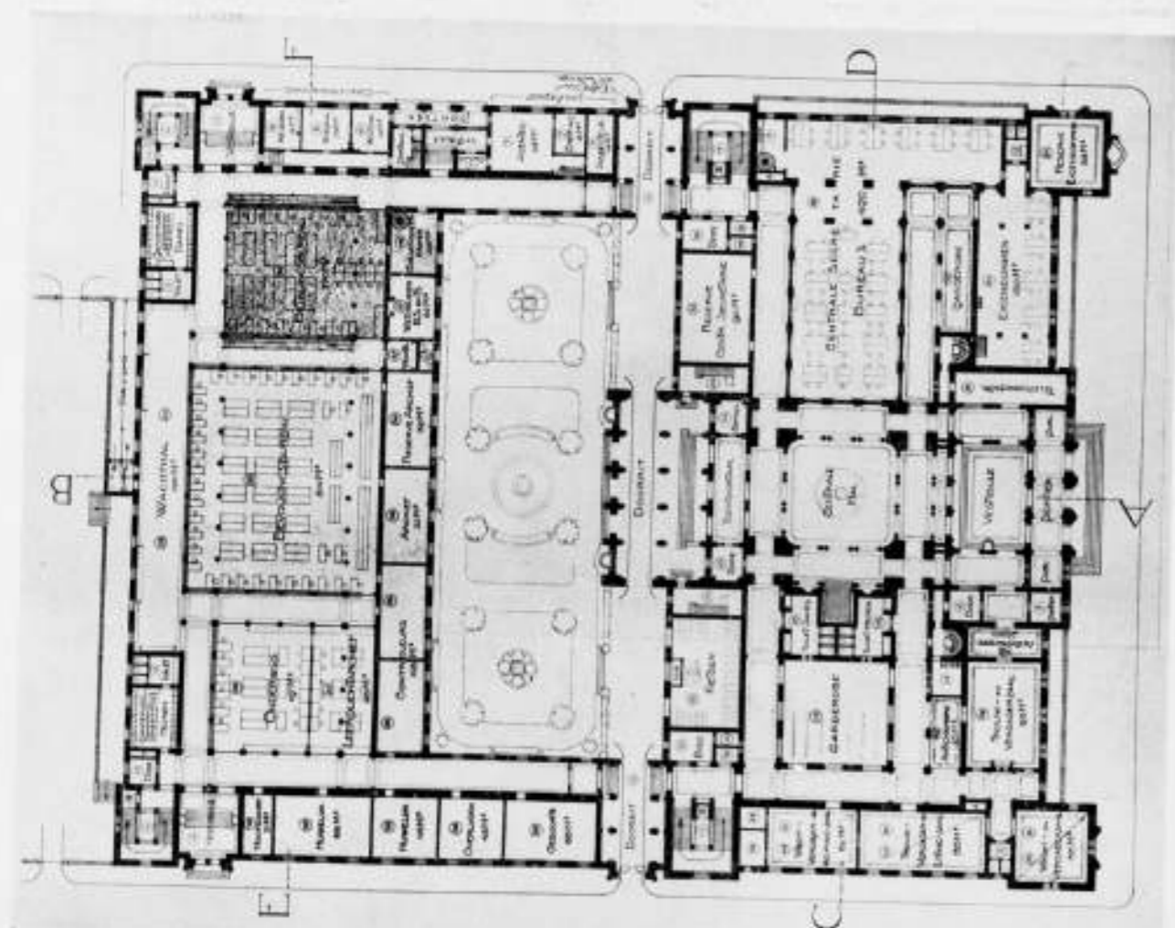
PRISVRAAG ROTTERDAMSCHE RAADHUIS. Ontwerp Motto: S. P. Q. R. van Prof. H. EVERS. Plan Begane grond. Schaal 1 op 720.
