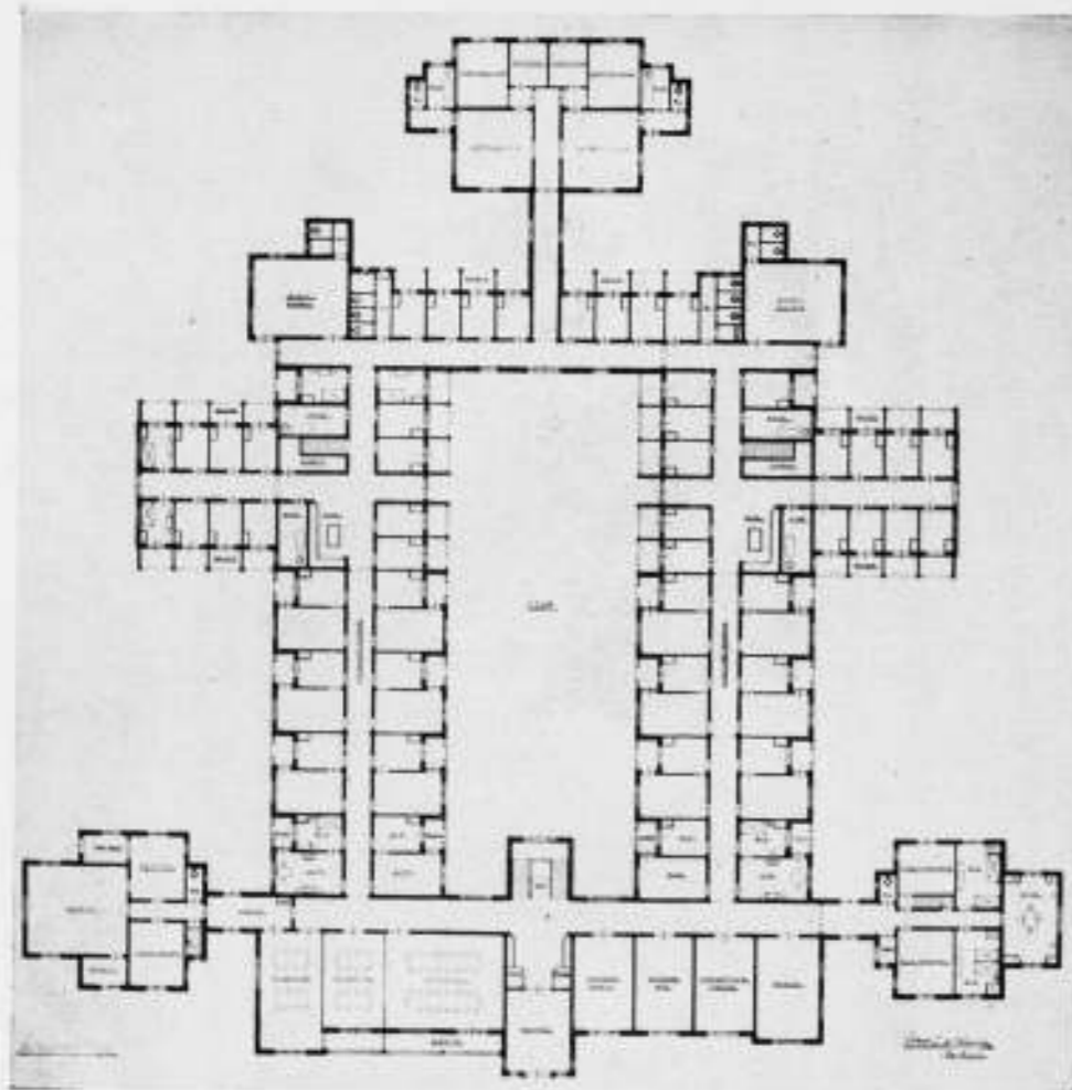
Te Huis voor alleenstaande blinden te Wolfhezen. Plan Beganegrond. Arch. Corns. L. de Koning.
