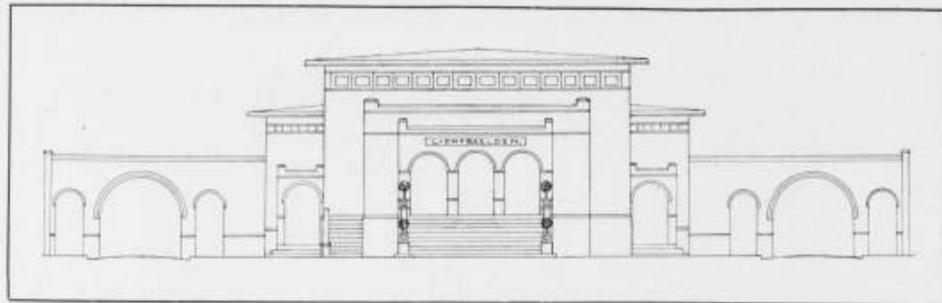
Tentoonstelling „Huis en Tuin” Hoofdgebouw: Theater en Restaurant. Voorgevel schaal 1 op 200.
