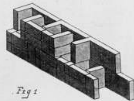
Afb. 4. De beton steenen, systeem „Schnell—Groffits”.
