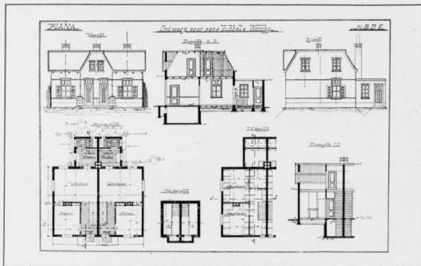
Woningtype A der N. B. D. S. te Gennep. Schaal 1 op 250.
