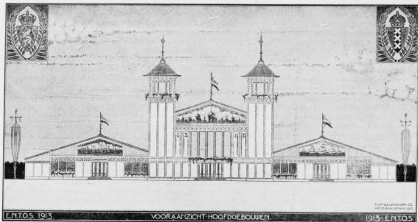
VOORAANZICHT VAN DE HOOFDGEBOUWEN DER EERSTE NEDERL. TENTOONSTELLING OP SCHEEPVAARTGEBIED Architect H. J. M. WALENKAMP Cz. Het complex van Hoofdgebouwen bestaat o. a. uit een Hoofdgebouw, waarvan wij hier het vooraanzicht geven, lang 112,5 M. en breed 62,5 M., waarachter om een binnenplaats van 65 M. bij 75 M. gegroepeerd zijn een machinegebouw, lang 45 M. en breed 25 M., en een galerijgebouw, diep 20 M. Spoedig hopen wij uitvoerig op dit onderwerp terug te komen.
