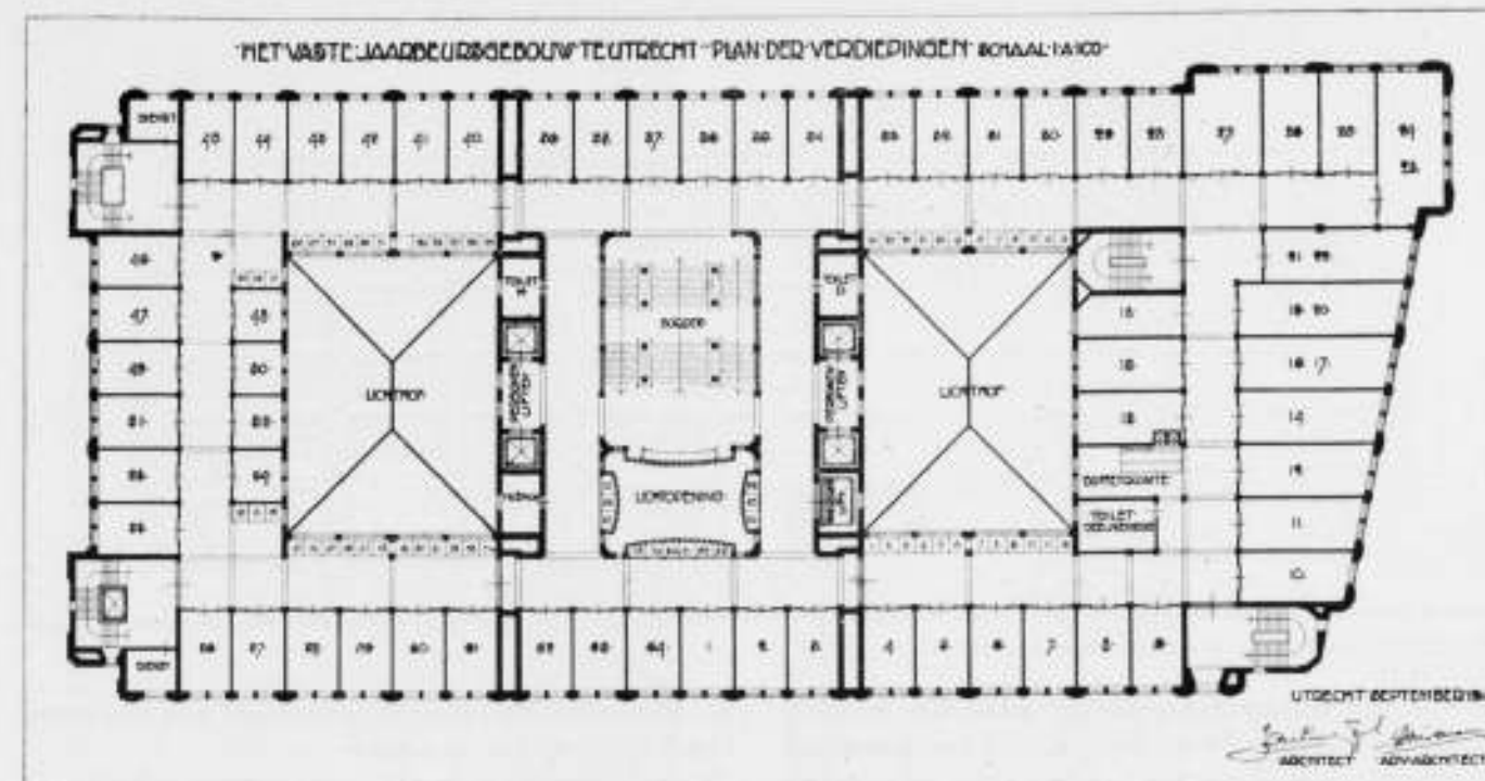
Het eerste Jaarbeursgebouw. Plan der verdiepingen.
