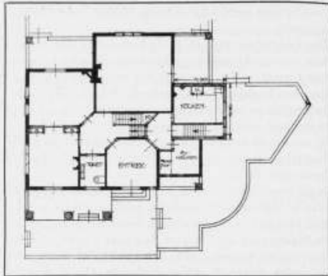
Fig. 1. Huije „Allegonda”. Plan beganegron. (Bestaand metselwerk is zwart aangegeven, nieuw metselwerk is gearceerd.)
