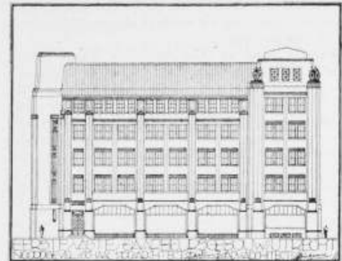
Het eerste Jaarbeursgebouw. Noordgevel.
