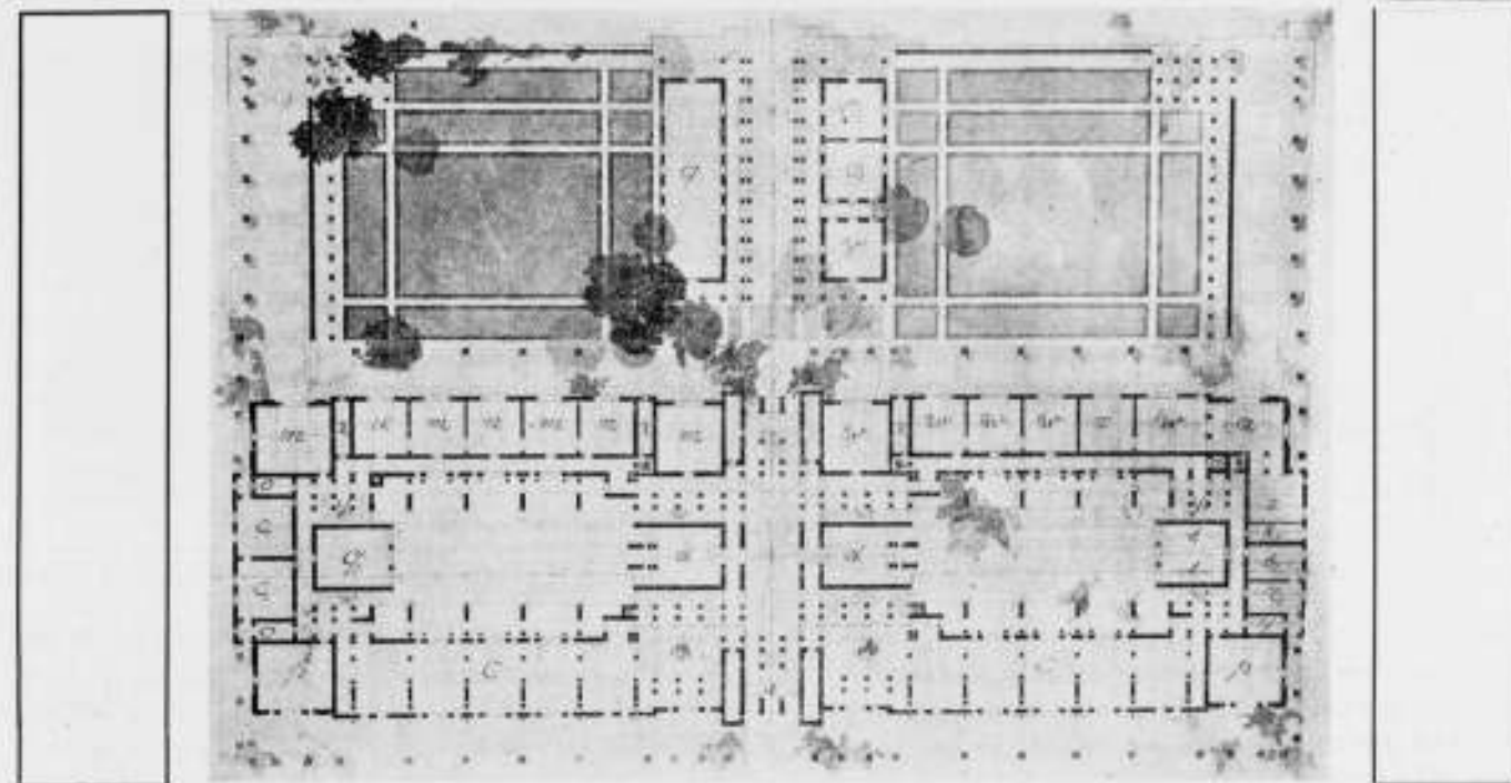
Fig. 1. Motto „Lage Landen“. 3e prijs.
