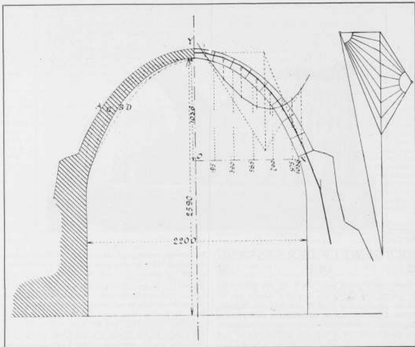
Fig. 2. A. Roadboog, B. Spitsboog, C. Ellips, D. Parabool.
