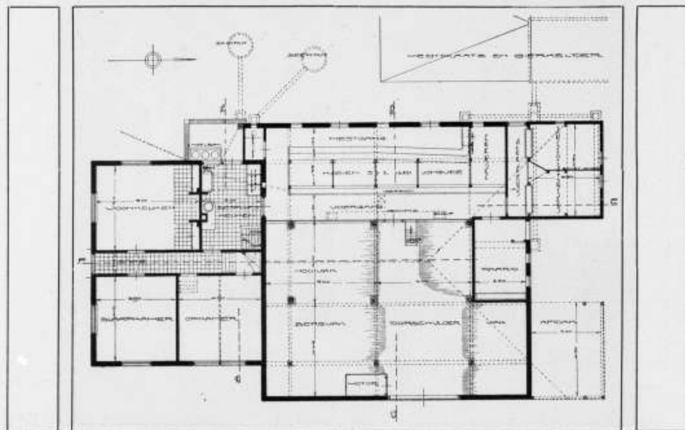
Ontwerp: „R.P.D.T.“ 4e prijs C. Plattegrond.
