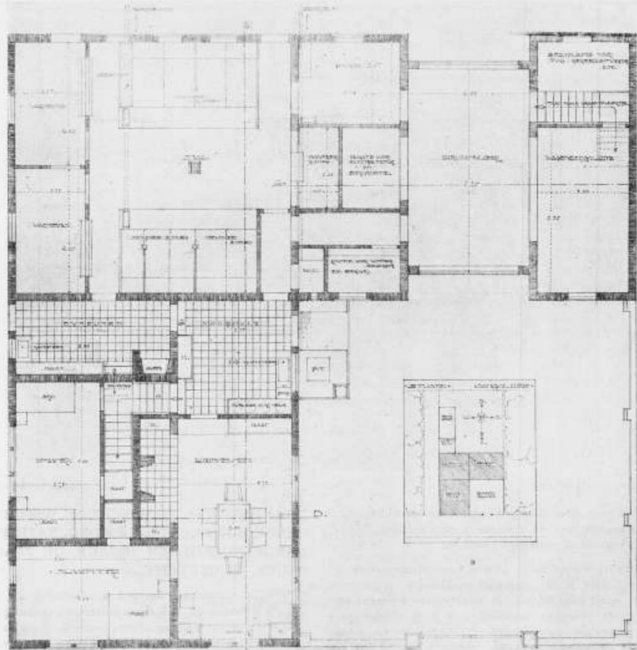
Ontwerp: III. Plattegrond.
