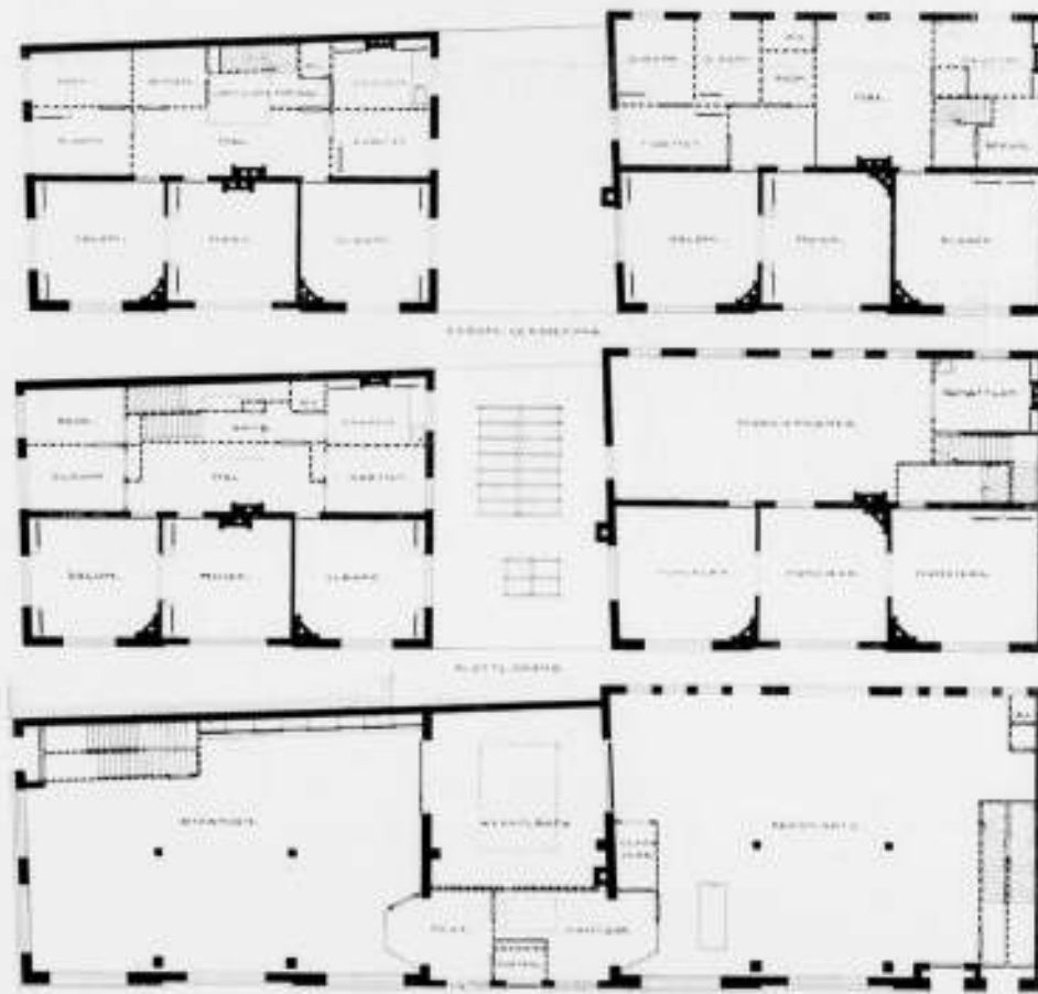
Auto garage en show-room te Den Haag.
