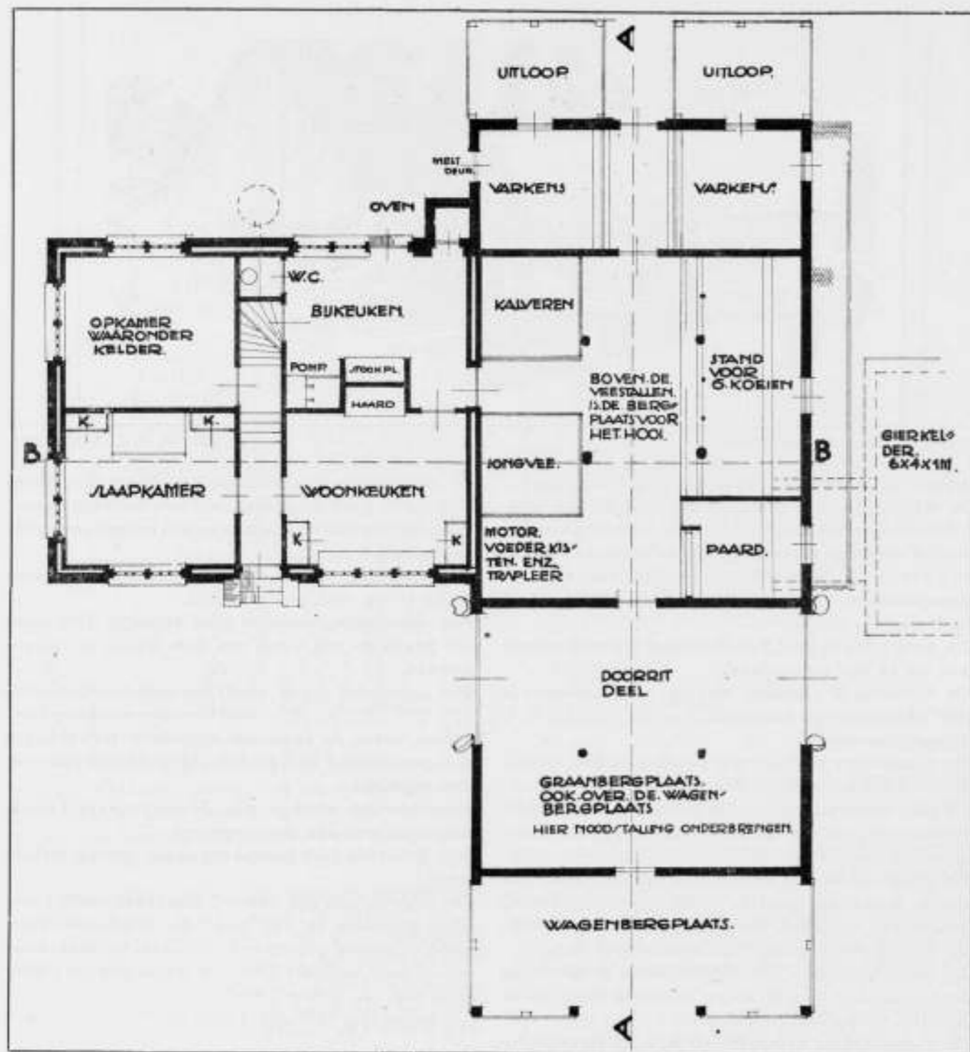
Ontwerp: „Beerengrauw”. 3e prijs. Plattegrond.
