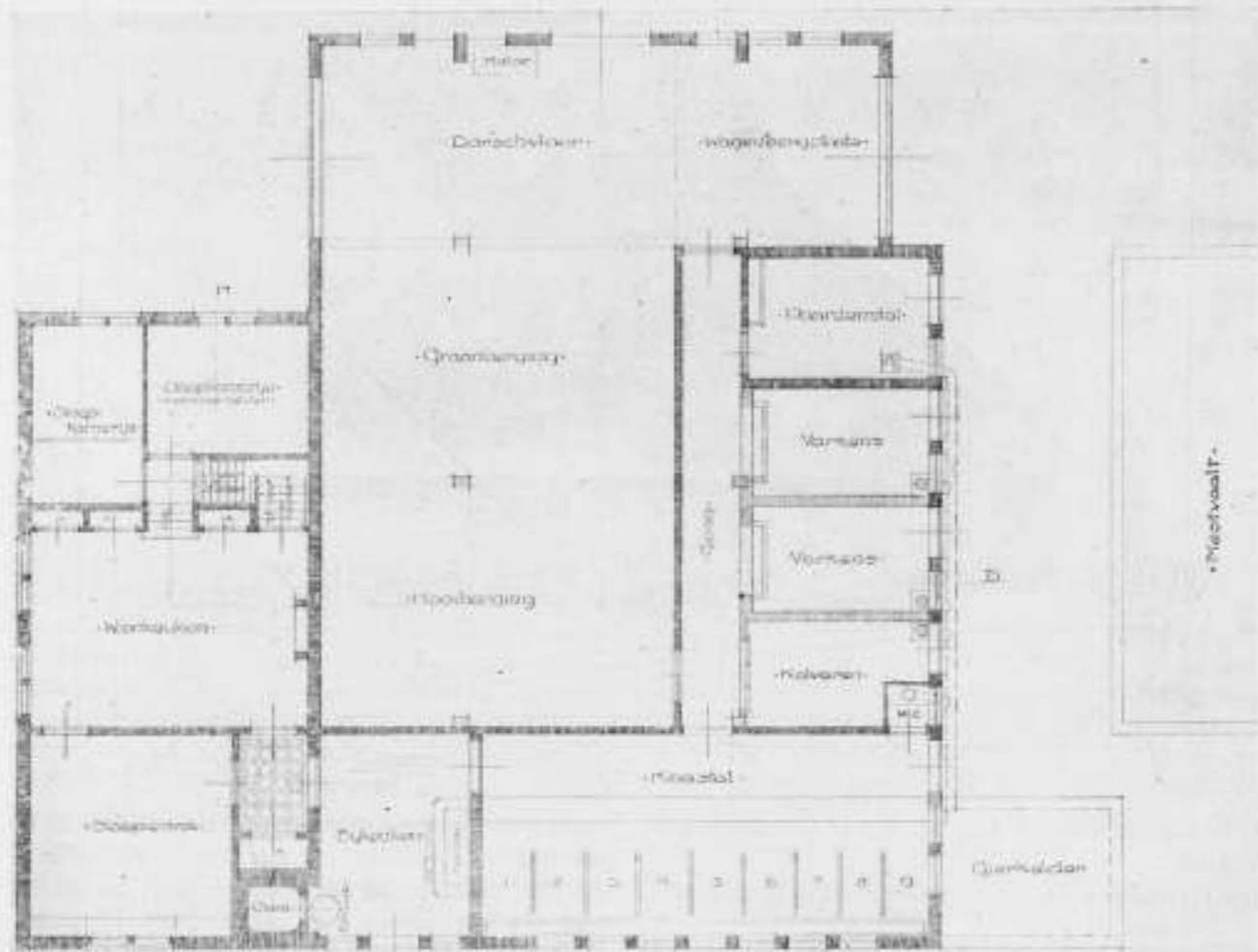
Ontwerp: „Friesland”. 2e prijs. Plattegrond.
