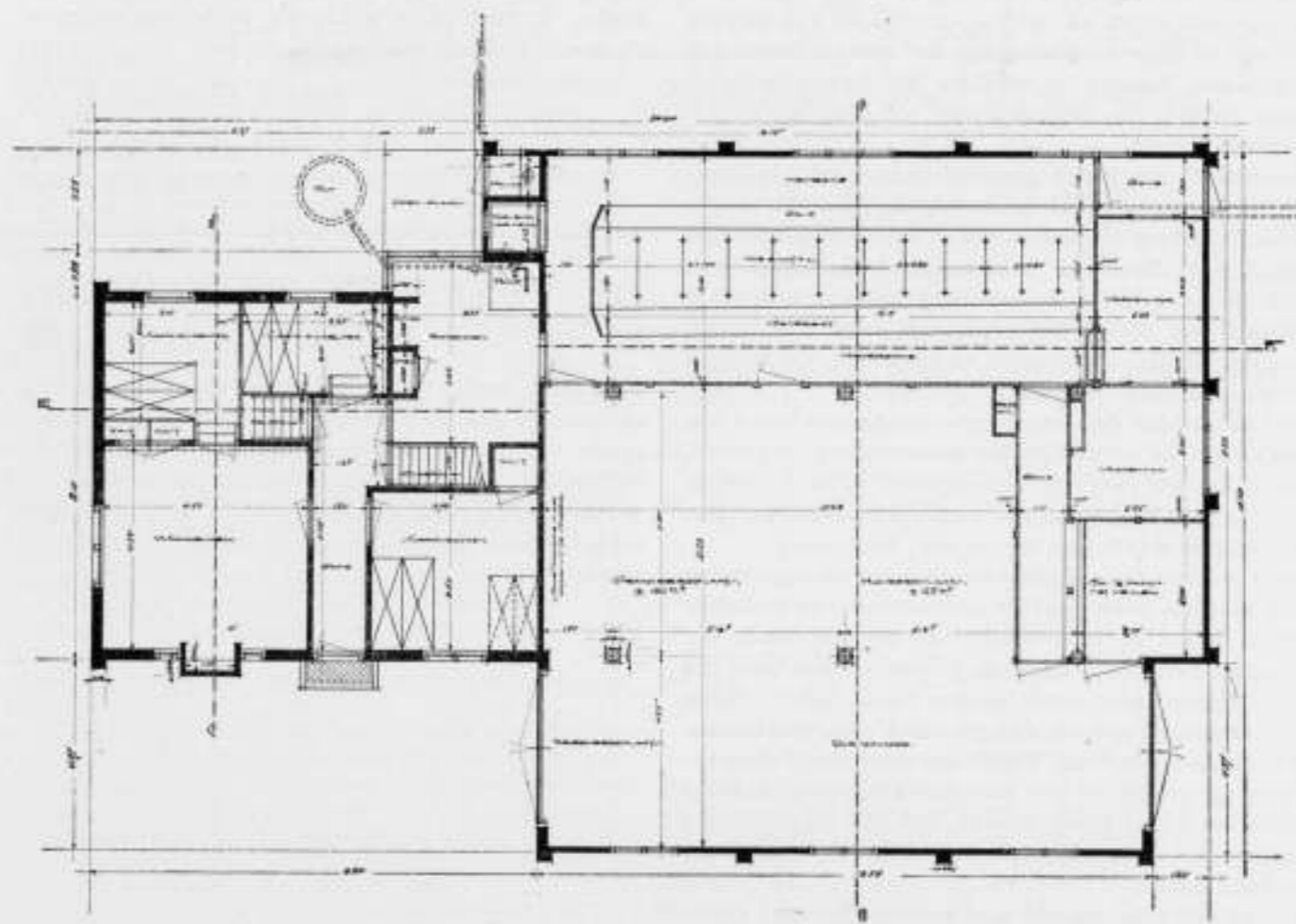
Ontwerp: „Rietdak”. 4e prijs B. Plattegrond.
