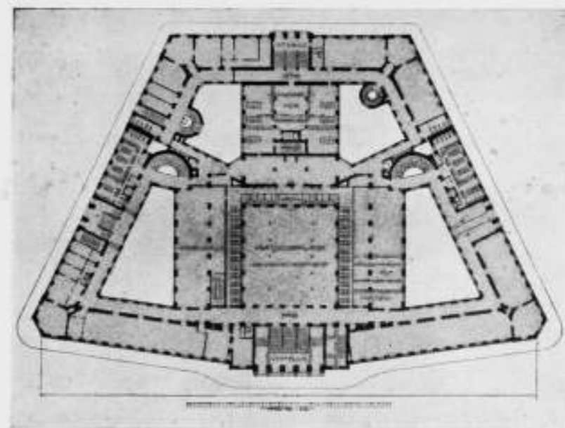
Postspaarbankgebouw te Weenen, Plattegrond.
