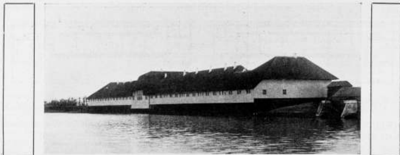
Fig. 3. Dubbele houten hulpschool aan den Zeeburgerdijk te Amsterdam.
