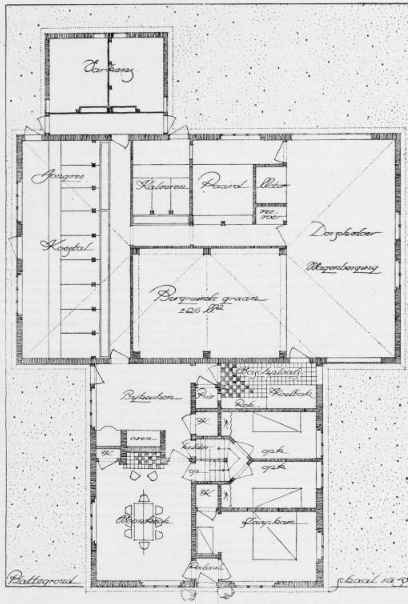
Ontwerp „Kultuur“, 1e prijs. Plattegrond.
