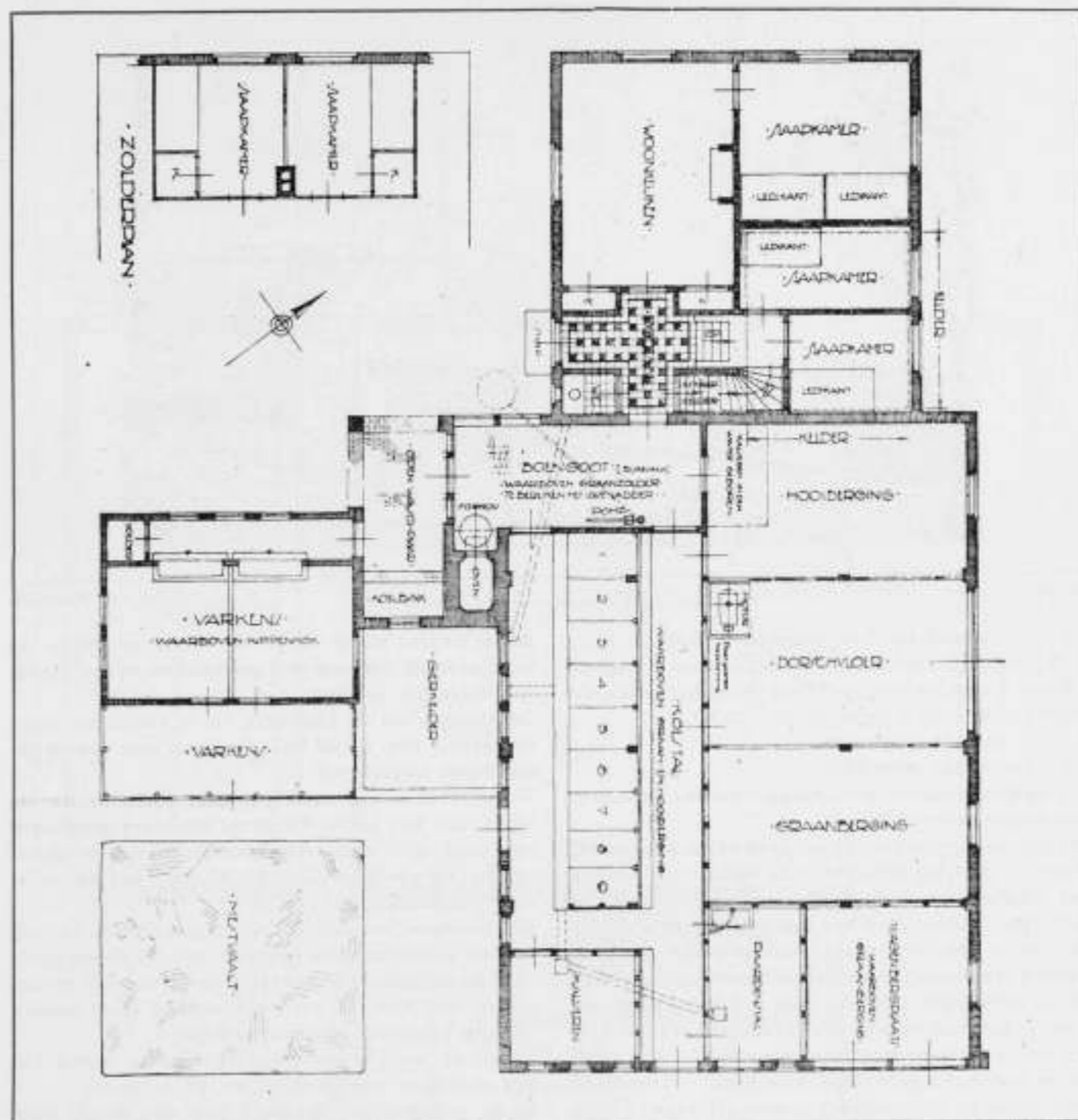
Ontwerp: „Zuid-Holland“. Plattegrond. 1e prijs.
