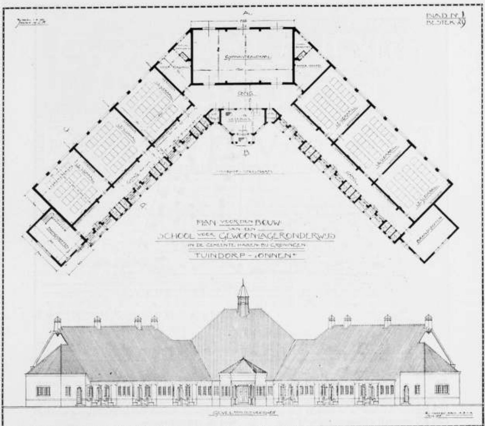
Ontwerp dorpschool te Haren.
