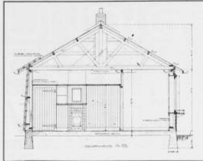
t Pannenhuis. Arch. J. C. v. Epen.
