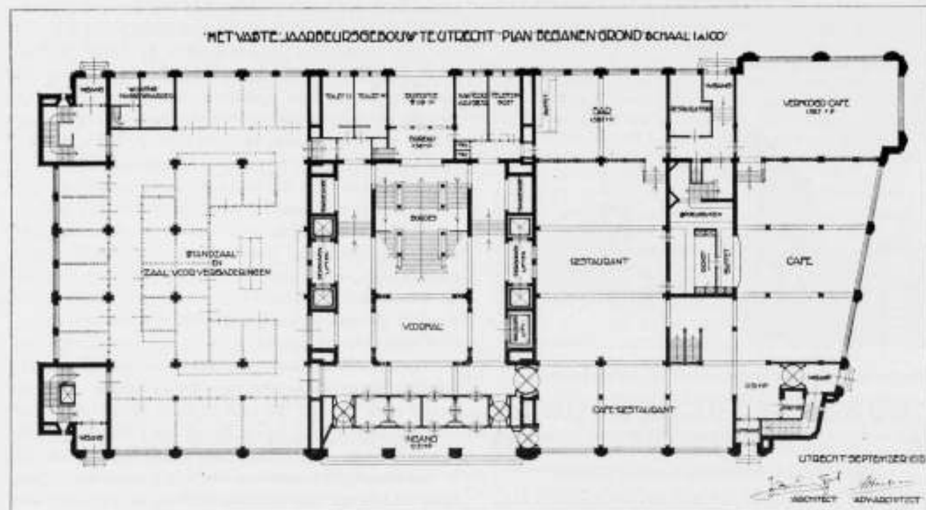
Het eerste Jaarbeursgebouw. Plan Begane Grond.
