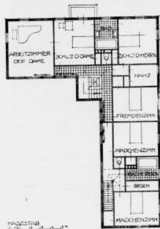
OBERGESCHOSS
