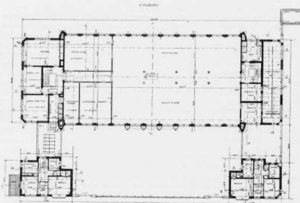
PLATTE GROND VERDIEPING. VIERDE TELEFOONCENTRALE AAN DEN MIDDENWEG IN DEN WATERGRAAFSMEER.
