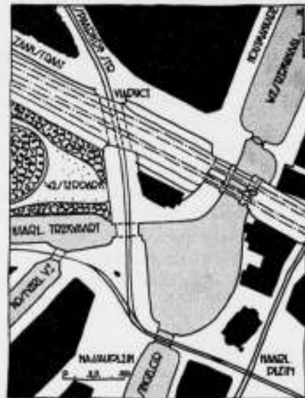
SITUATIE, VIADUCT BIJ DE SPAARNDAMMERSTRAAT.
