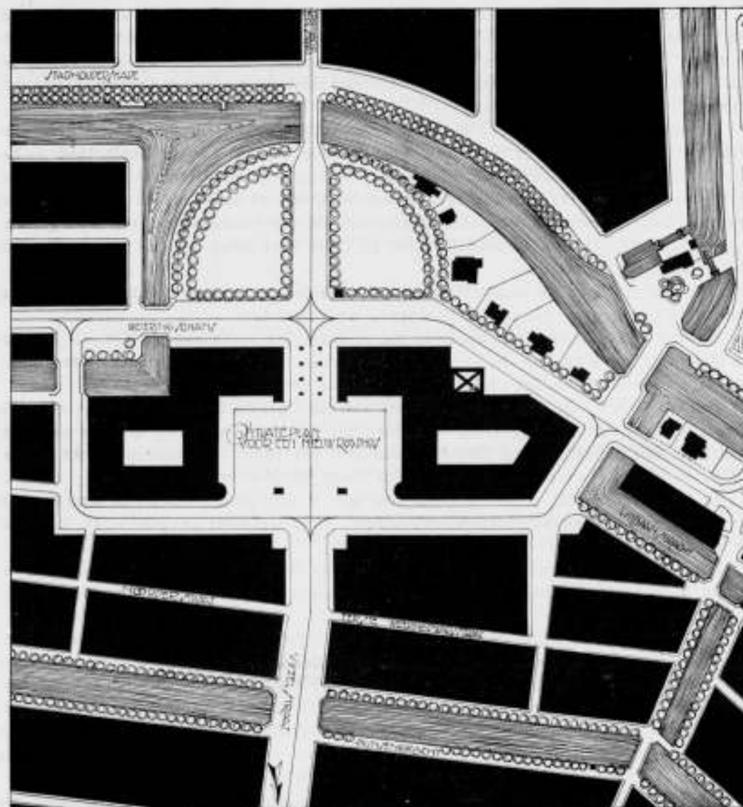
SITUATIEPLAN, OP DEZELFDE HOOFDGEDACHTTE GEBASEERD, DOCH MEY DAARIN AANGERRACHTTE WIJZIGINGEN.
