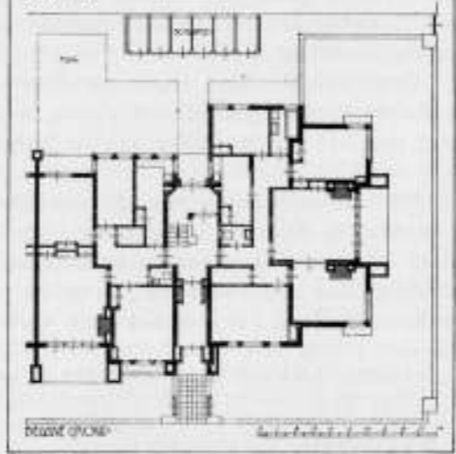
WONINGGROEP „DAAL EN BERG“ TE 'S-GRAVENHAGE. JAN WILS, ARCHITECT.
