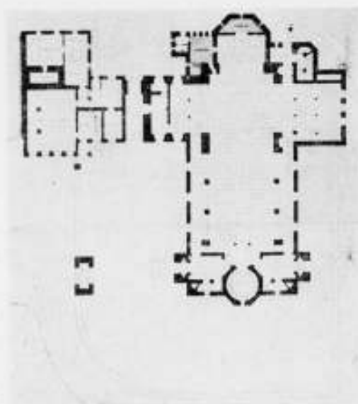
MÅSTUGGSKERK TE GÖTEBORG.
