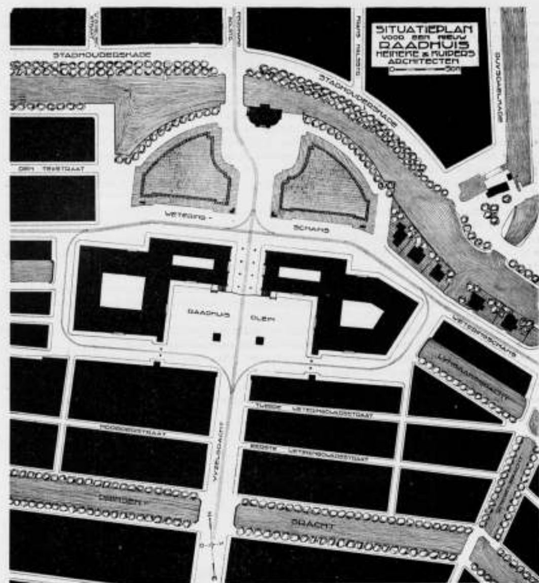
SITUATIEPLAN VOOR EEN NIEUW RAADHUIS TE AMSTERDAM, ARCHITECTEN HEINEKE EN KUIPERS.
