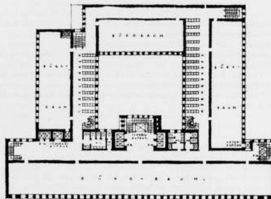
PRIJSVRAAG VOOR EEN ONTWERP VOOR EEN KANTOORGEBOUW TE DÜSSELDORF. MOTTO: „RHEINLAND“. ONTWERP PROF. PETER BEHRENS.
