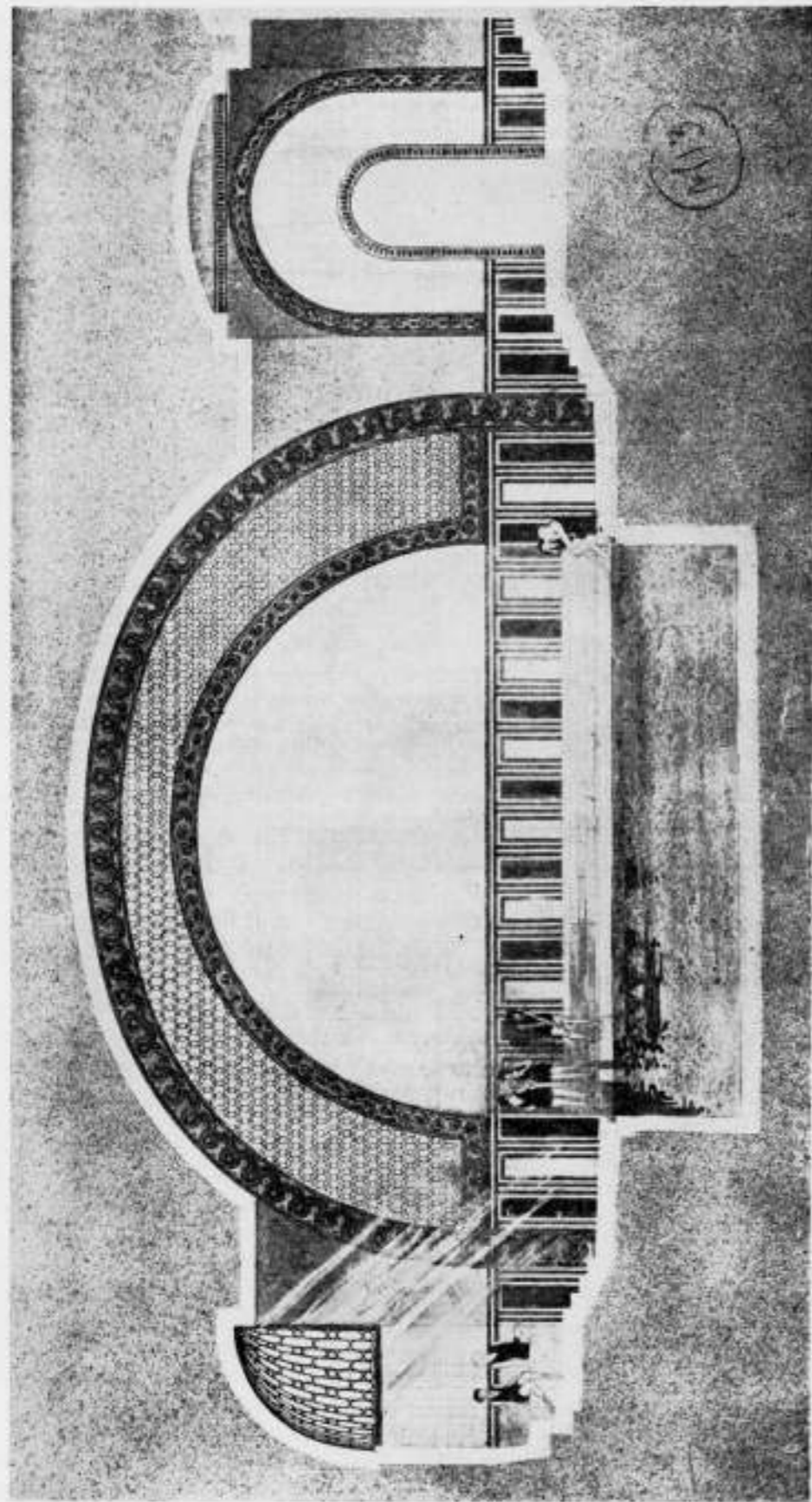
ONTWERP VOOR EEN BADHUIS. DOORSNEDE OVER HET BASSIN
