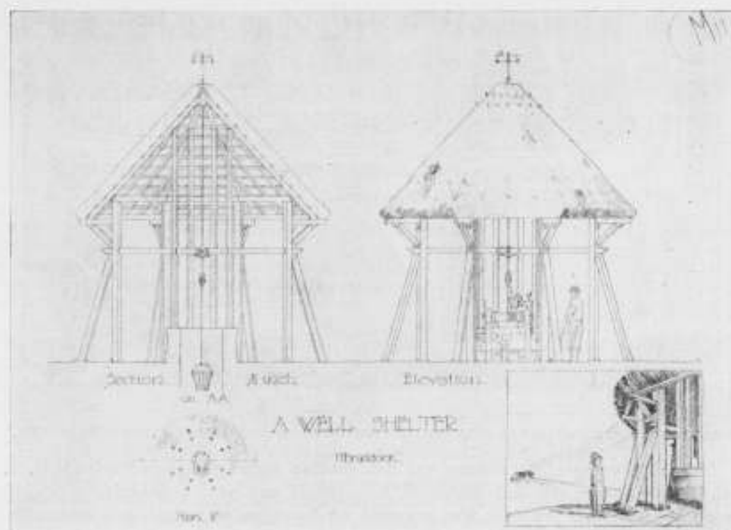
EEN AFDAKJE BOVEN EEN PUT.
