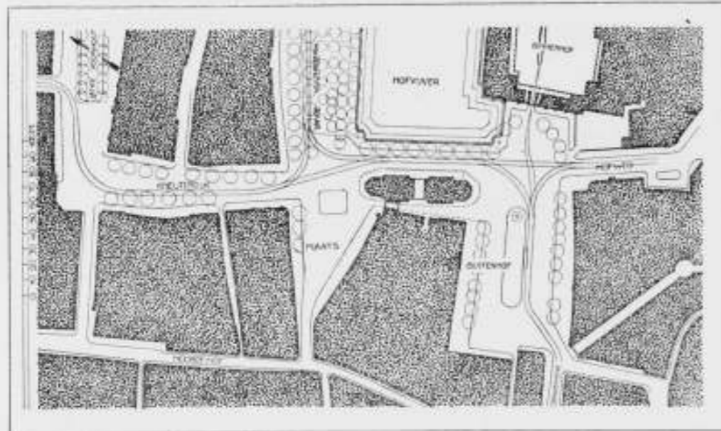
SITUATIE VAN DEN VERKEERSWEG TUSSEN KNEUTERDIJK EN BUIJENHOF VOLGENS HET ONTWERP 1921.
