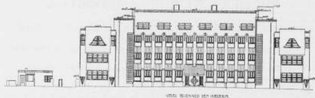
KANTOORGEBOUW TEN BEHOEVE VAN DE GEMEENTETRAN TE AMSTERDAM. PLATTEGRONDEN 1E EN 2E VERDIEPING EN VOORGEVEL.
