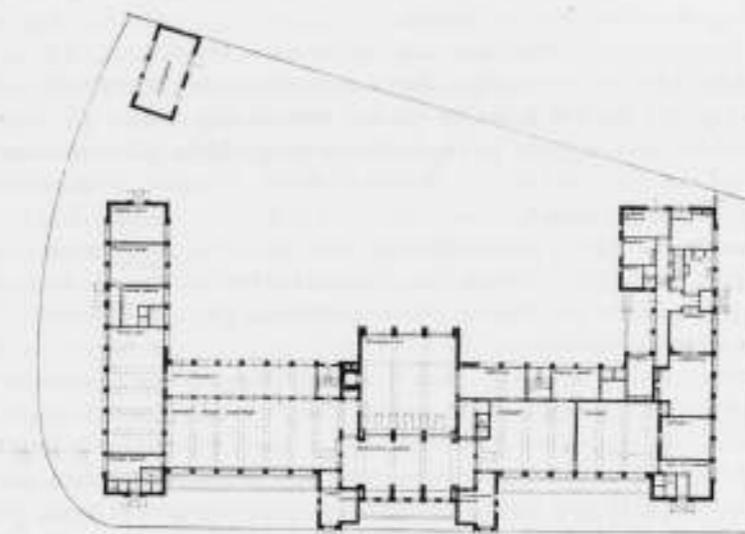
POST- EN TELEGRAAFKANTOOR TE SITTARD. ONTWERP IR. G. FRIEDHOFF.
