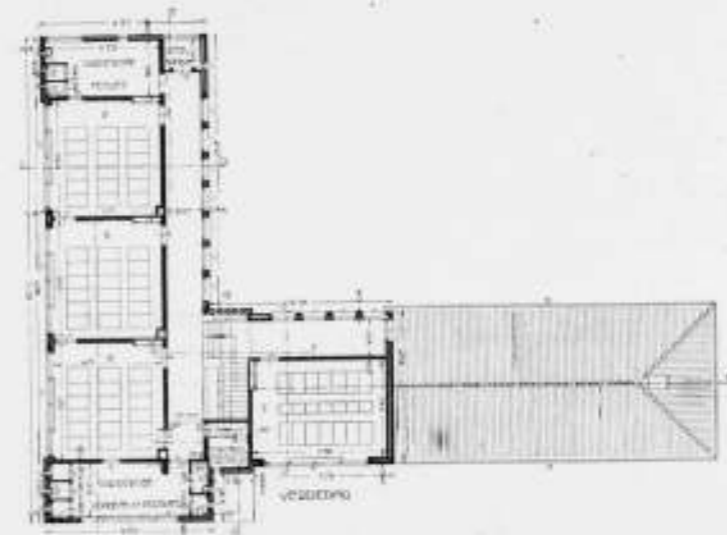
PLATTEGROND VAN DE SCHOOL AAN HET LAVENDELPLEIN TE HILVERSUM. W. M. DUDOK. Architect.
