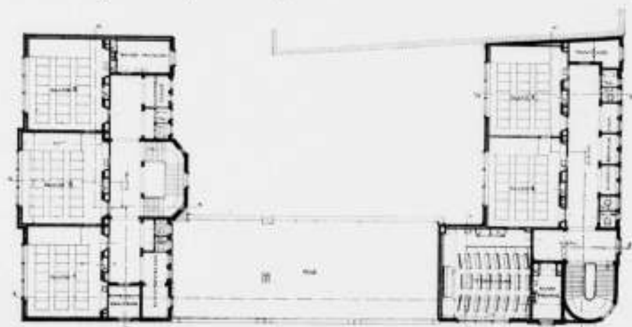
PLATTEGROND DUBBELE SCHOOL AAN DE OUDE SCHANS.
