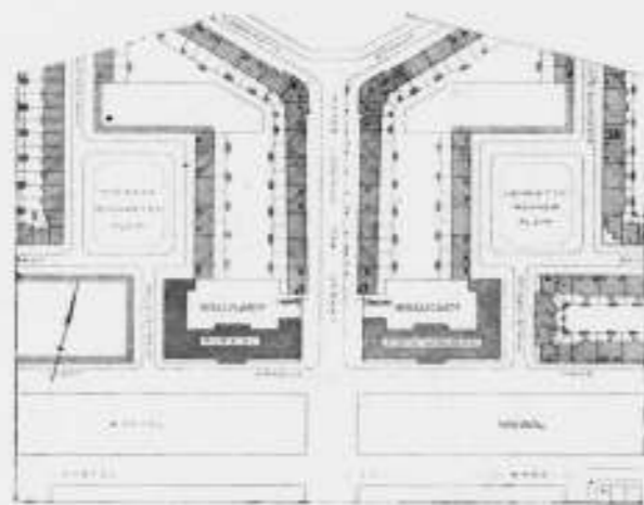
SITUATIE VAN DE SCHOOLGEBOUWEN AAN DE JOZEF ISRAËLSKADE TE AMSTERDAM.
