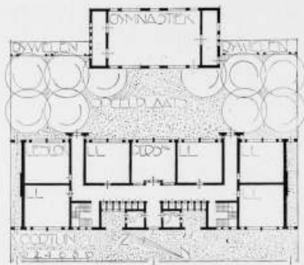
R. K. SCHOOL TE 'S-GRAVENHAGE ARCH. Ir. J. KLIJNEN. PLAN BEGANE-GRONDVERDIEPING.
