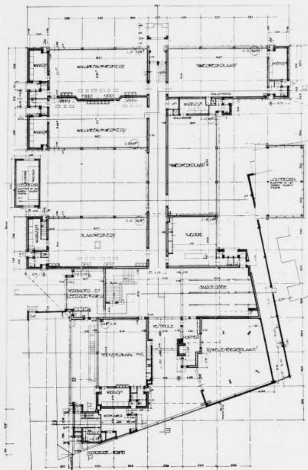
PLAN DERDE AMBACHTSSCHOOL TE 'S-GRAVENHAGE.
