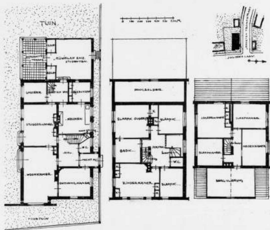
PLATTEGRONDEN EN SITUATIE VAN HET WOONHUIS AAN DE JULIANALAAN TE DELFT. Architect Ir. J. KLIJNEN B.N.A.
