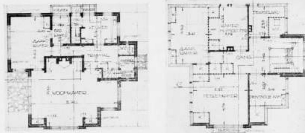
PLATTEGRONDEN VAN HET LANDHUIS TE WASSENAAR.
