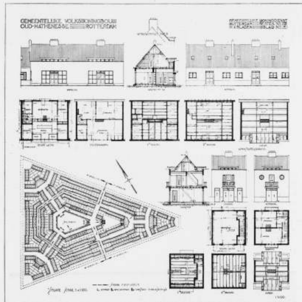
GEM. WONINGBOUW. SITUATIE, TYPE D (WINKEL) ARCHITECT „OUD MATHENESSE” TE ROTTERDAM. EN ADMINISTRATIEGEBOUWTJE. J. J. P. OUD.
