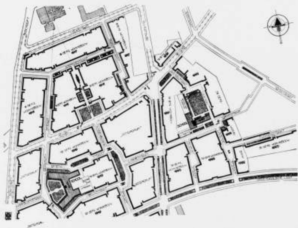
SITUATIEPLAN VAN HET LAVENDELPLEIN EN OMGEVING TE HILVERSUM.
