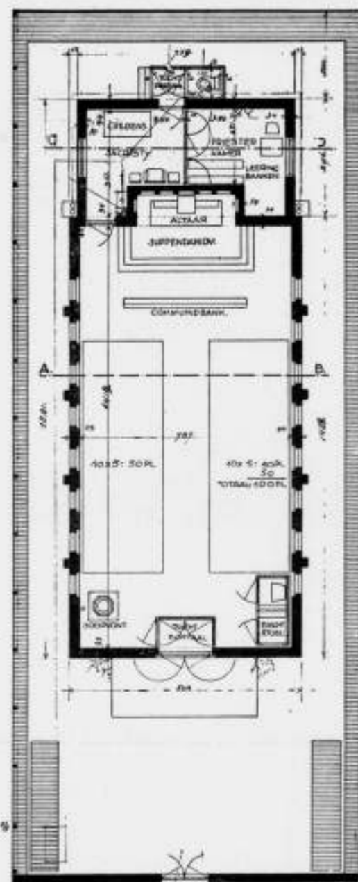
R. K. KAPEL TE PAPENDRECHT. H. P. J. DE VRIES, Architect.
