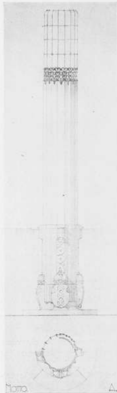
MOTTO A. Eerste Prijs. Aanzicht bij dag. PRIJSVRAAG MONUMENTALE LANTAARNS OP DEN DAM TE AMSTERDAM.
