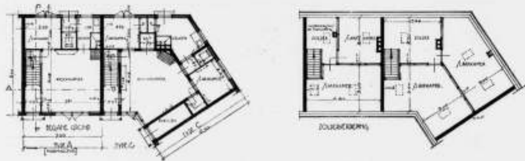
GEM. WONINGBOUW TE ROTTERDAM ARCHITECT „OUD MATHENESSE“ TYPE A (NORMAAL TYPE) C (EEN DER HOEKTYPEN) J. J. P. OUD.
