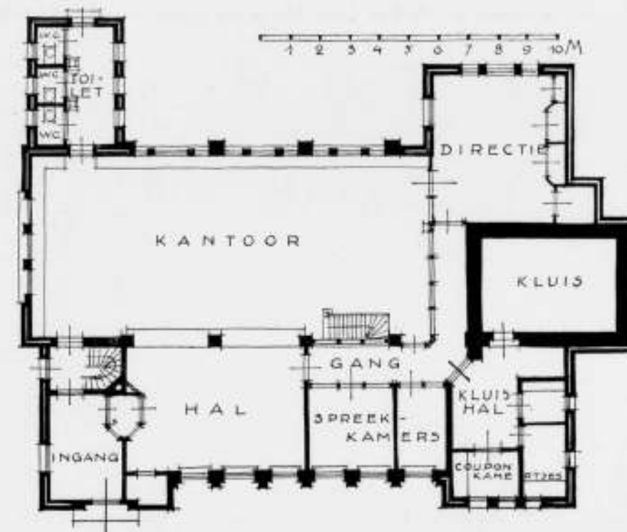
KANTOORGEBOUW VAN DE NATIONALE BANKVEREENIGING TE ASSEN. ARCHITECT Ir. H. F. MERTENS, B. N. A.
