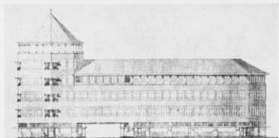
Motto: K.K.K. Inzending onder het Motto: K.K.K. voorgedragen voor een geldelijke beloning van f 400.— ROKIN-PRIJSVRAAG TE AMSTERDAM.
