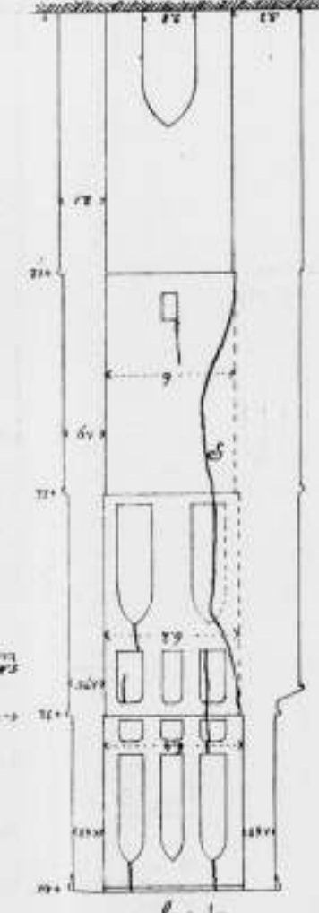
Fig. 4. Standgicht volgens cd op fig. 2
