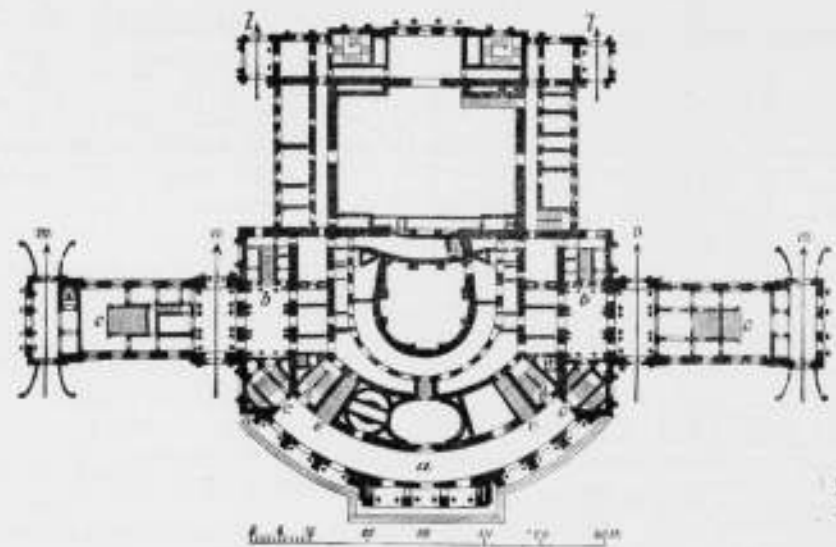
Platen grond van den nieuwen hofschouwburg te Weenen.
