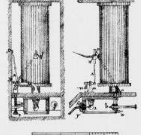
Fig. 13. Condensator met Ontlader
